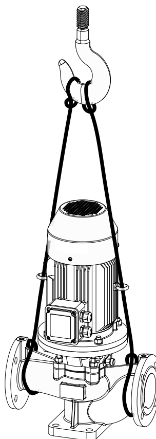
Перемещение насосов Rz-L с рым-болтами
