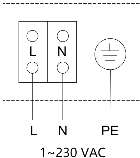
Схема подключения однофазного асинхронного электродвигателя 1~230 VAC
