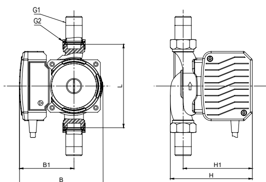
Габаритные размеры насоса Rz-MP20-3-6
