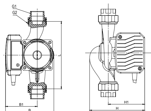
Габаритные размеры насоса Rz-MP25-7-8 Rz-MP32-9-12
