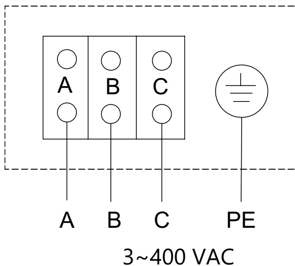
Схема подключения трехфазного асинхронного электродвигателя 3~400 VAC
