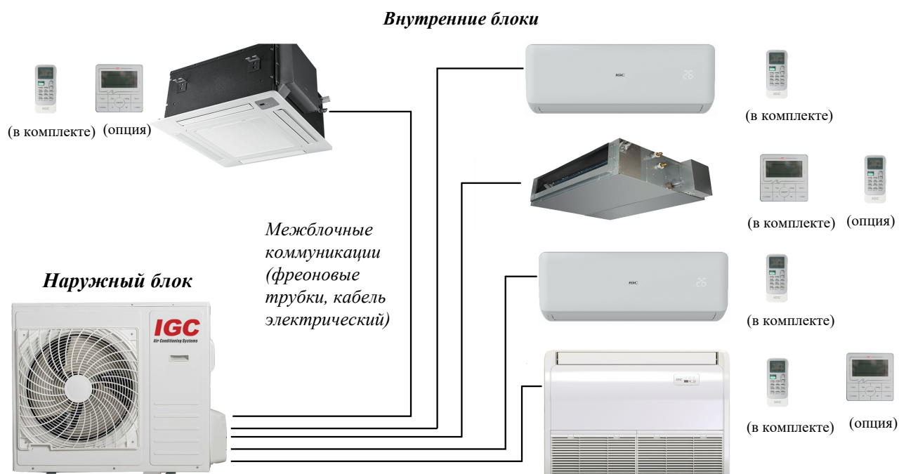
Рис.1- Состав мульти сплит-системы IGC
