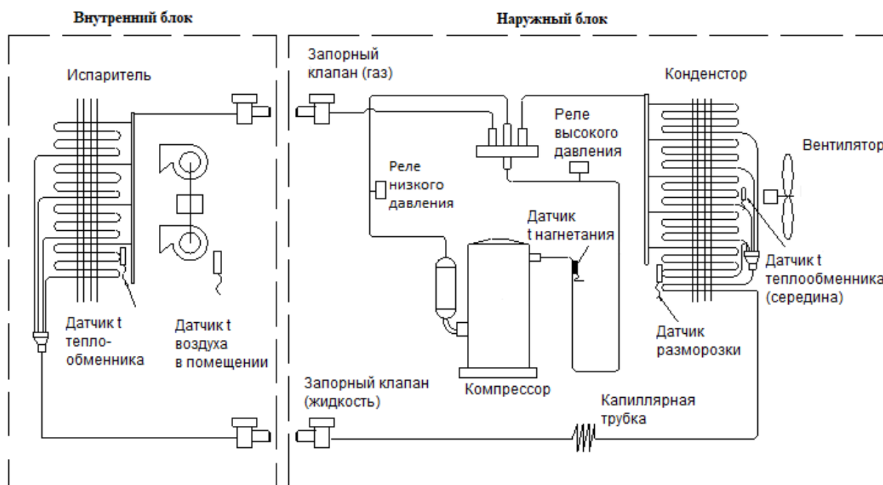
Рис.2 -Фреоновый контур кондиционера
