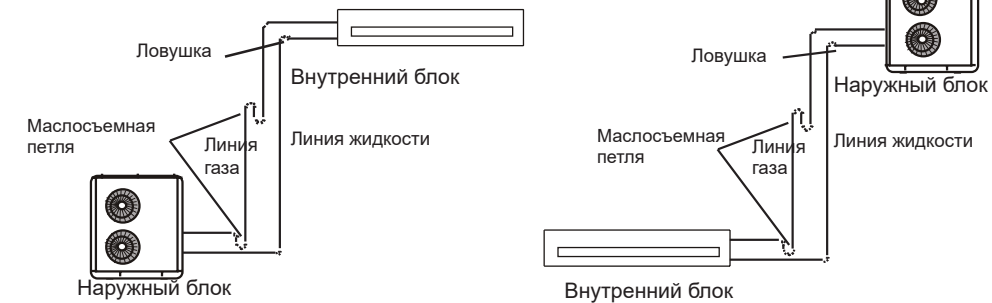
Внутренний блок установлен выше наружного.
