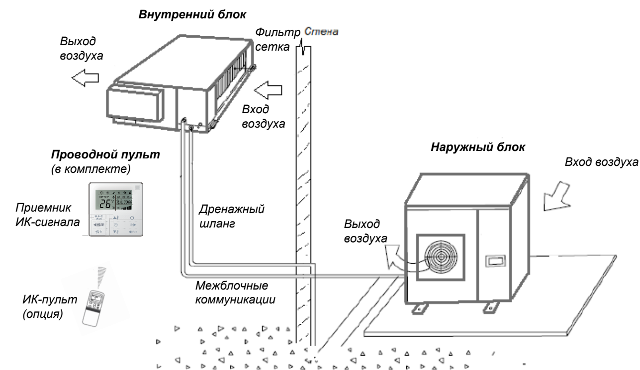
Рис.1 -Состав кондиционера
