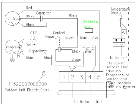
Наружный блок моделей RAS/RAC-24AX,30AX,36AX
