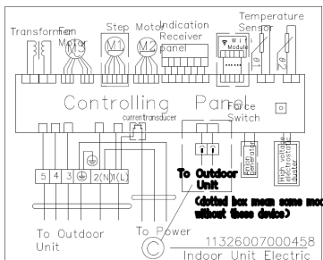
Внутренний блок моделей RAS/RAC-24AX, 30AX, 36AX
