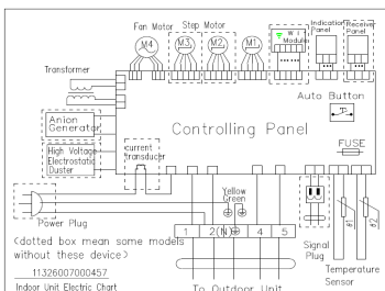
Внутренний блок моделей RAS/RAC-12AX, 18AX
