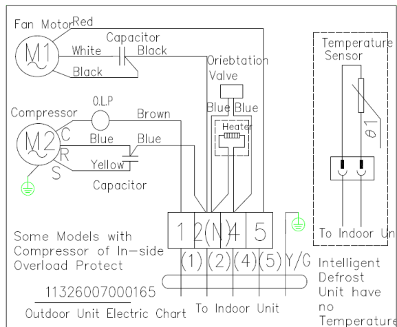
Наружный блок моделей RAS/RAC-07AX,09AX,12AX,18AX
