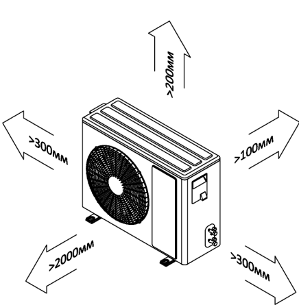
Установочные размеры наружных блоков
