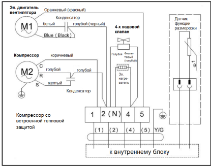
Схема электрическая наружных блоков
