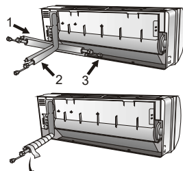
Возможные направления прокладки трубопровода
