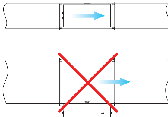
Рисунок 5.3 – Варианты монтажа
