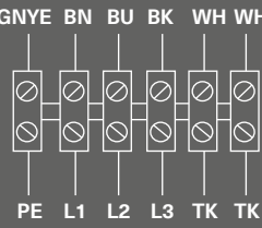
Схема 5 (400 В, 3 ф.)
