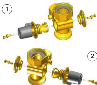
Рис. 7: Трёхходовой смешивательный клапан (1 - подача справа; 2 - подача слева)
