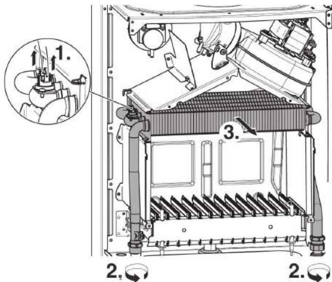
Рис. 27 Чистка теплообменника
