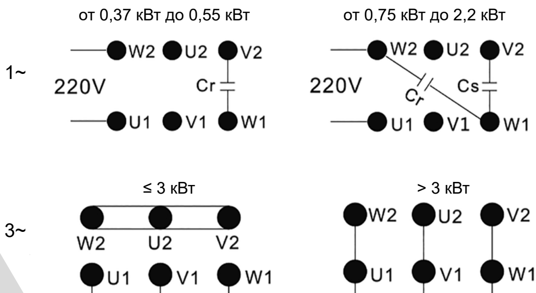
Рисунок 4. Схема электроподключения
