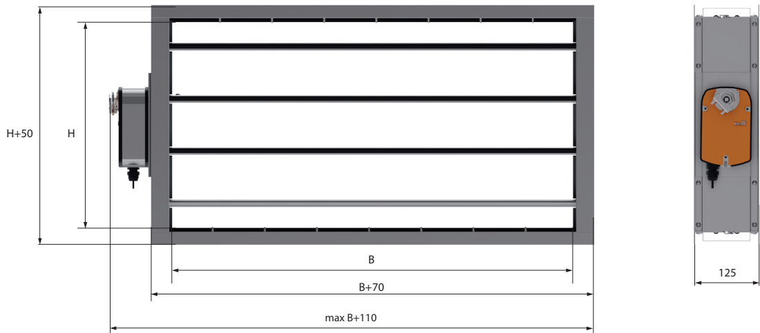
Габариты (мм) и масса (кг) клапанов SRA*
