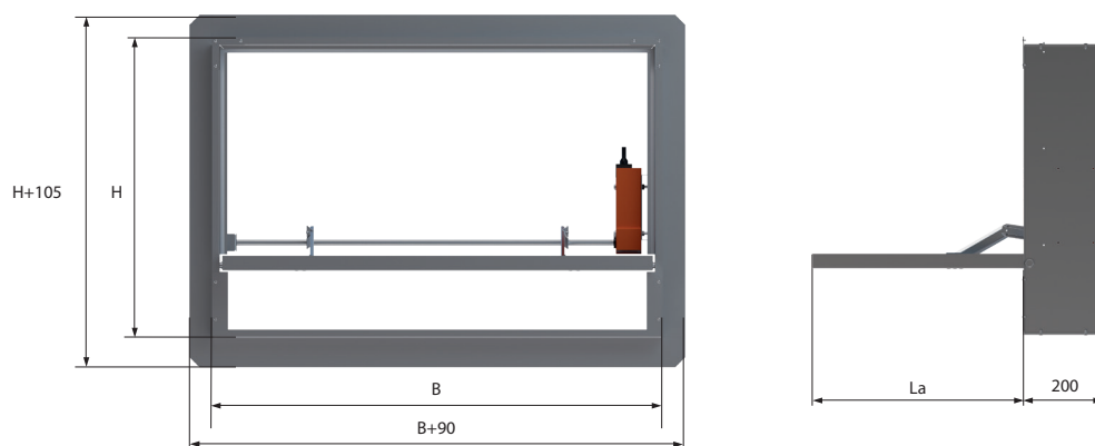
Габариты (мм) и масса (кг) клапанов DVSW Е 90 и 180
