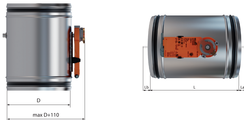
Характеристики AGRJ
