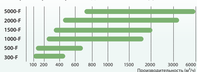
Типоразмеры и производительность ОТД-E
