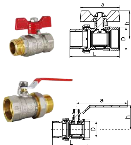
Кран шаровый латунный со сгоном (американка) ВР-НР
