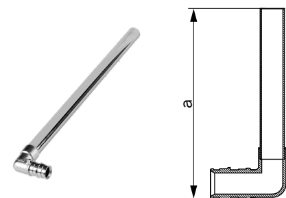
Трубка L-образная d 15 для подключения радиатора
