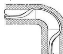
Проход с внешней стороны колена
