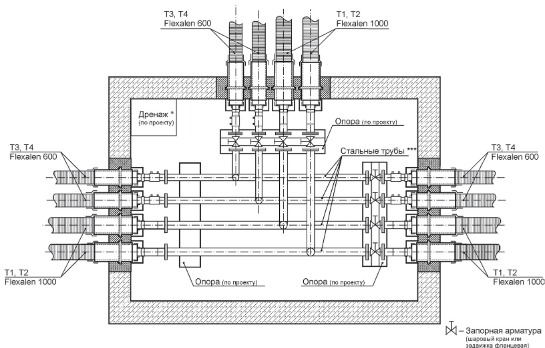
Пример устройства ответвлений при прокладке двух трубопроводов (схематично)
