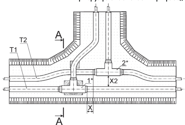
Пример устройства ответвлений при прокладке двух трубопроводов (схематично)
