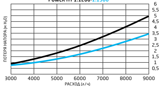
ХАРАКТЕРИСТИКА РАСХОД-НАПОР ДЛЯ КОТЛОВ POWER HT 1.450-1.650-1.850-1.1000-1.1200-1.1500
