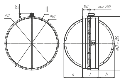
Рисунок 9 — Исполнение с лючком D ≥ 1120
