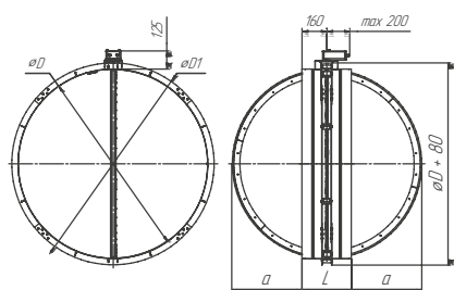
Рисунок 7 — Ниппельное исполнение D \geq 1120
