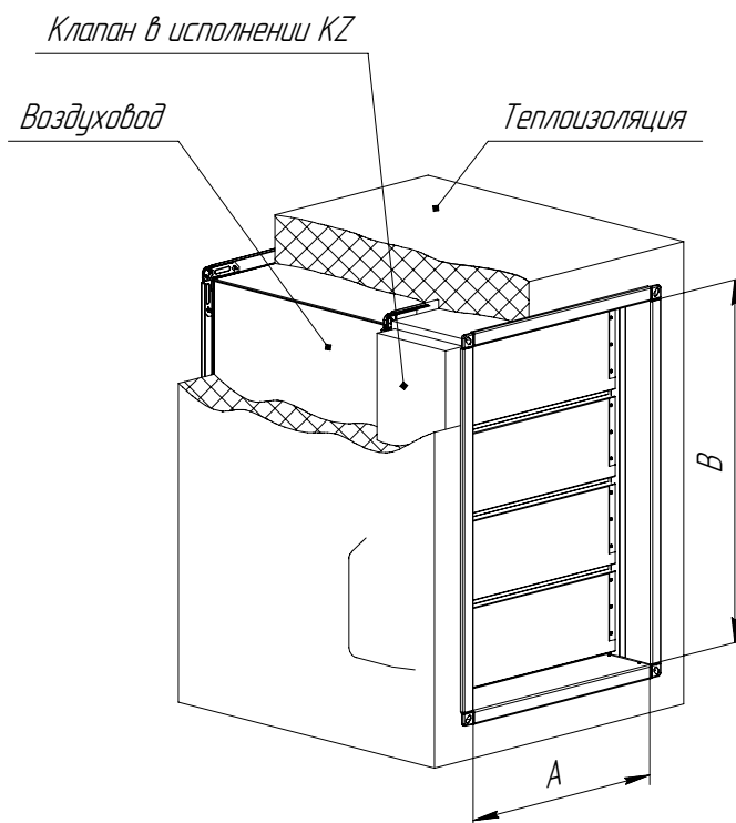
Клапан KD ML канальный с электромеханическим приводом снаружи
