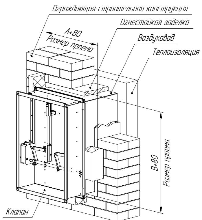
Клапан КД канальный с электромеханическим приводом внутри
