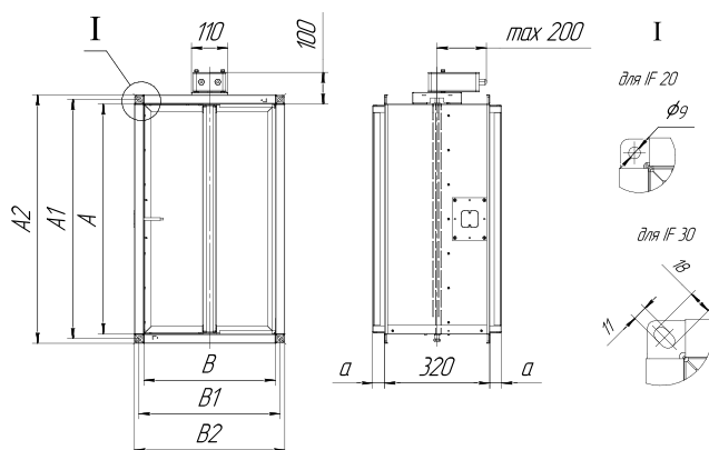
Рисунок 1 — Исполнение 04 без кожуха
