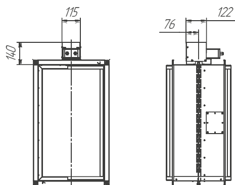
Рисунок 1 — Исполнение без кожуха
