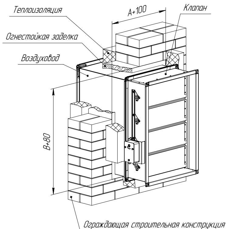
Клапан КД МЛ каналный с электромеханическим приводом снаружи
