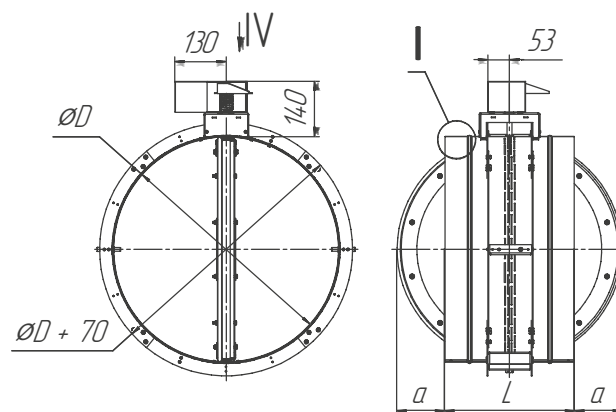
Рисунок 4 — Ниппельное исполнение 500 \leq D \leq 1000
