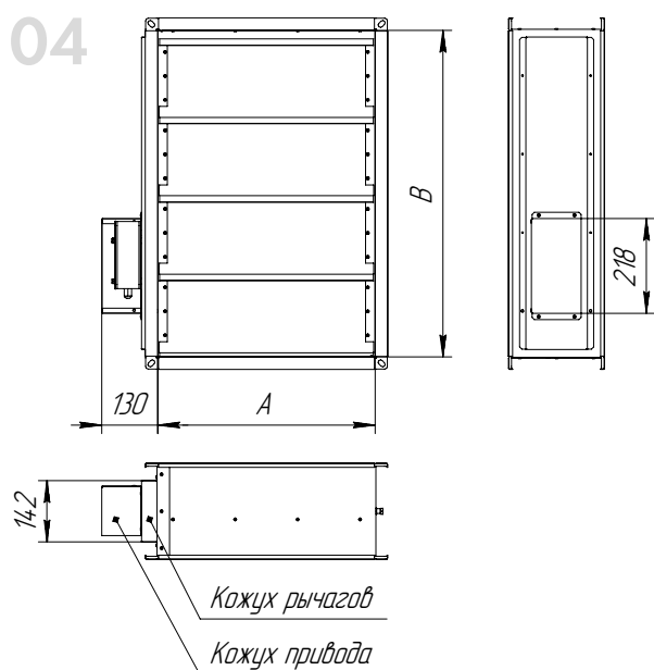
Исполнение 04 с KZ
