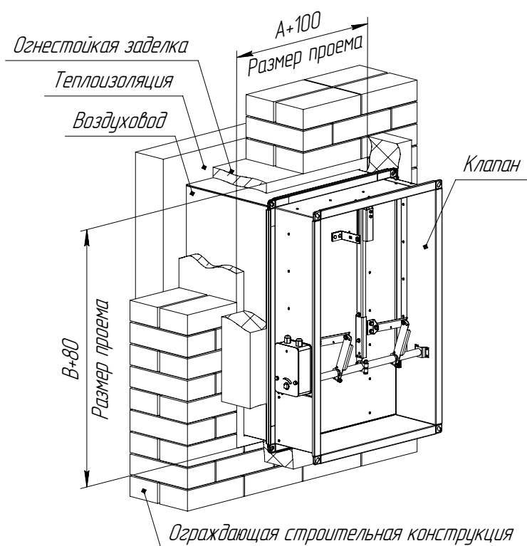
Клапан KD каналный с электромеханическим приводом снаружи
