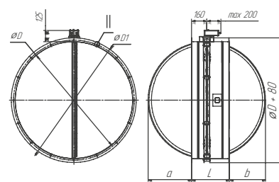
Рисунок 9 — Исполнение с лючком D \geq 1120
