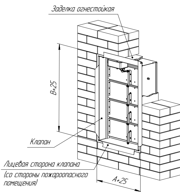
Клапан КД МЛ стеновой с электромеханическим приводом
