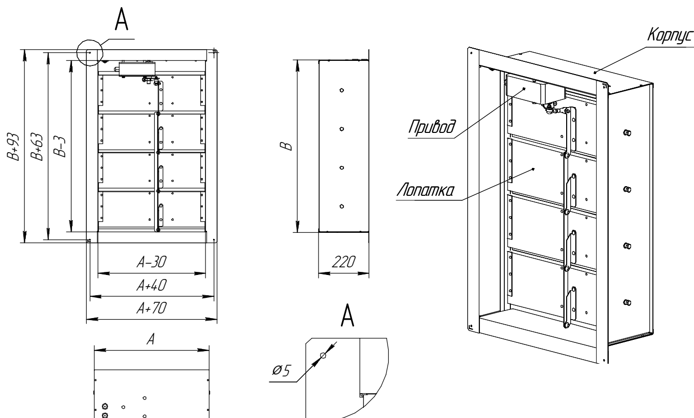
Клапан KPNZ-90-F1-VN-MN-ML, исполнение 04
