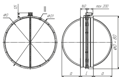
Рисунок 8 — Фланцевое исполнение D \geq 1120
