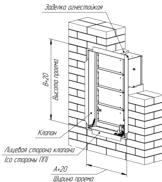
Клапан КД МЛ стеновой с электромагнитным приводом
