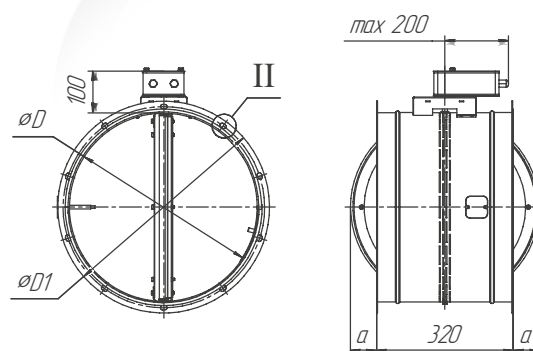
Рисунок 2 — Фланцевое исполнение D \leq 450
