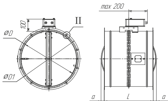
Рисунок 3 — Исполнение с лючком D \leq 450
