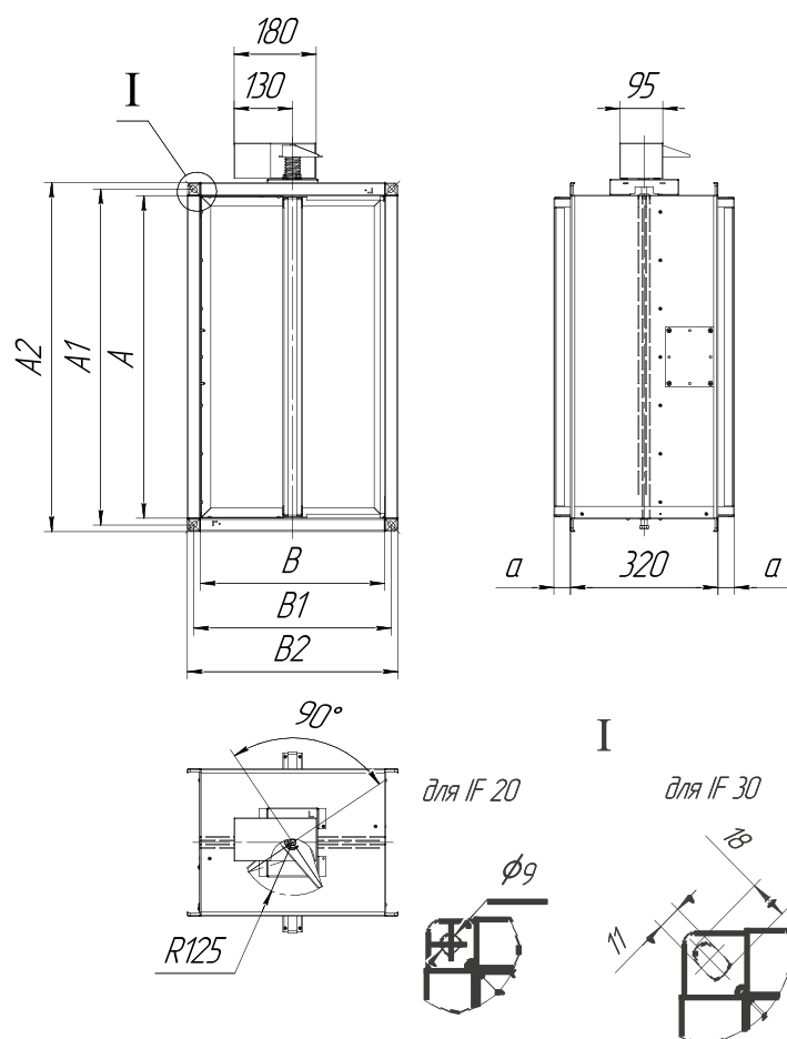
Рисунок 1 — Исполнение 04 с электромагнитным приводом
