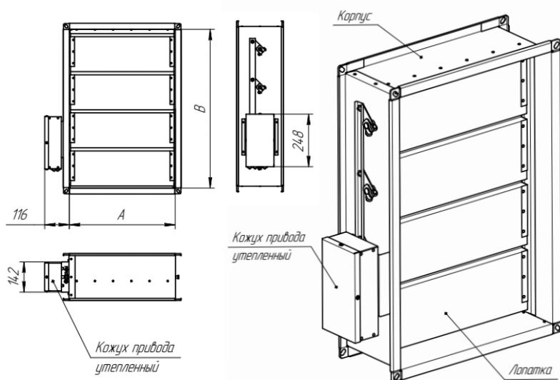
Клапан KPNZ-90-F2-SN-MN-ML, исполнение 12
