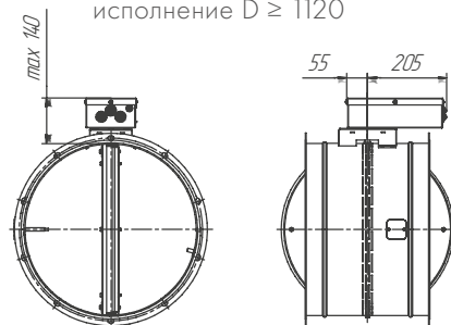
Рисунок 11 — Исполнение 12 с защитным кожухом, остальные размеры см. рисунки 1-9
