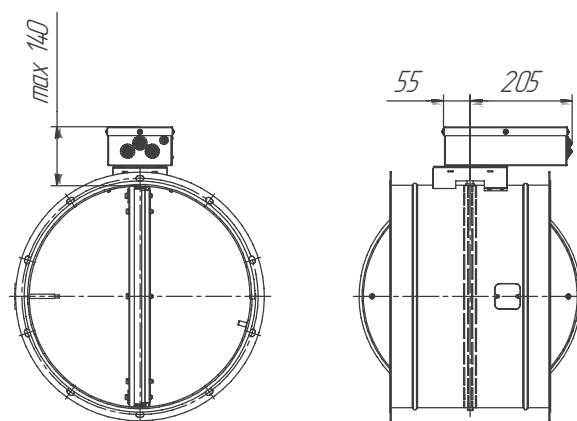
Рисунок 11 — Исполнение 12 с защитным кожухом, остальные размеры см. рисунок 1-9
