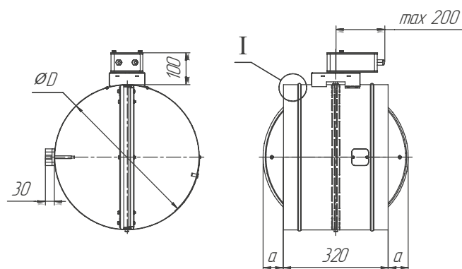
Рисунок 1 — Ниппельное исполнение D \leq 450
