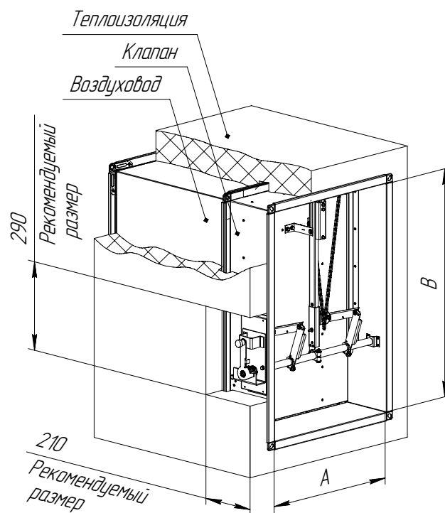
Клапан KD канальный с электромагнитным приводом снаружи
