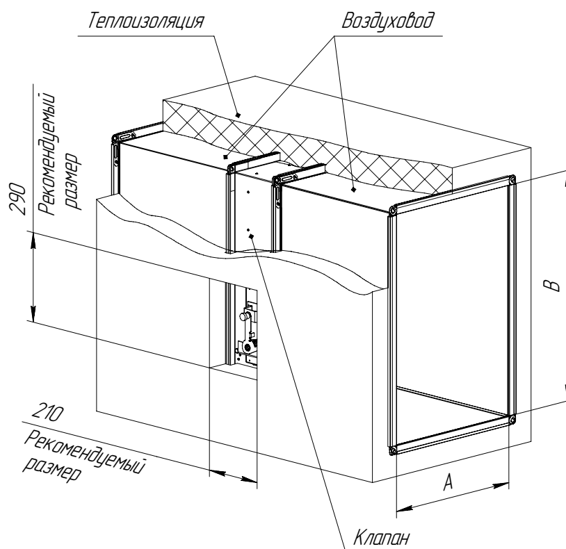
Клапан KD канальный с электромагнитным приводом снаружи
