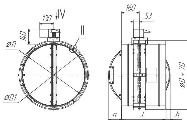
Рисунок 6 — Исполнение с лючком 500 \leq D \leq 1000
