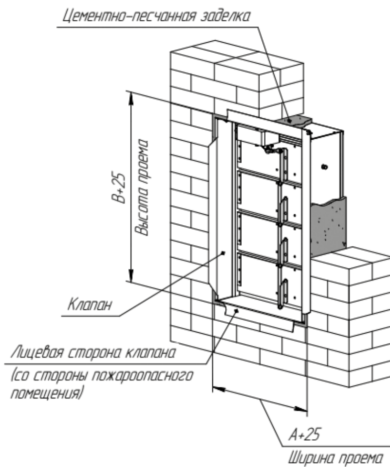
Клапан KPNZ ML стеновой с электромеханическим приводом
