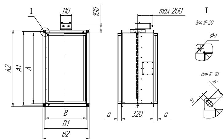
Рисунок 1 — Исполнение без кожуха
