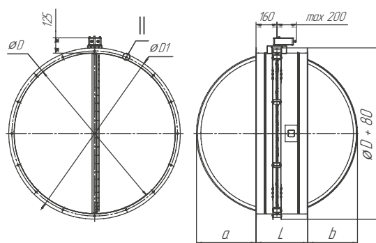
Рисунок 9 — Исполнение с лючком D \geq 1120
