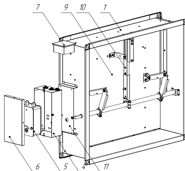
Конструкция клапана KD с приводом MN
