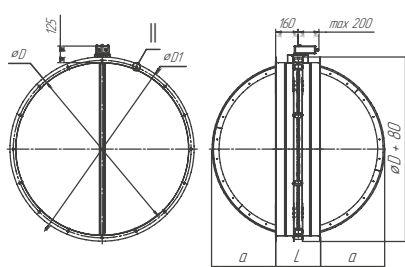
Рисунок 8 — Фланцевое исполнение D \geq 1120
