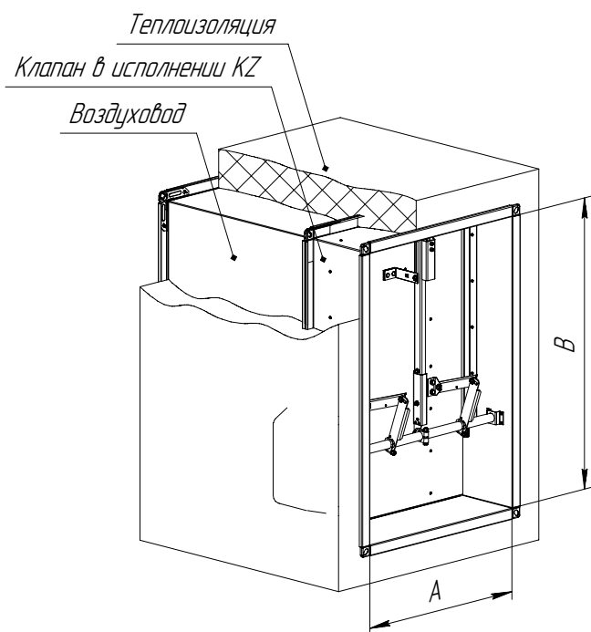
Клапан KD канальный с электромеханическим приводом снаружи
