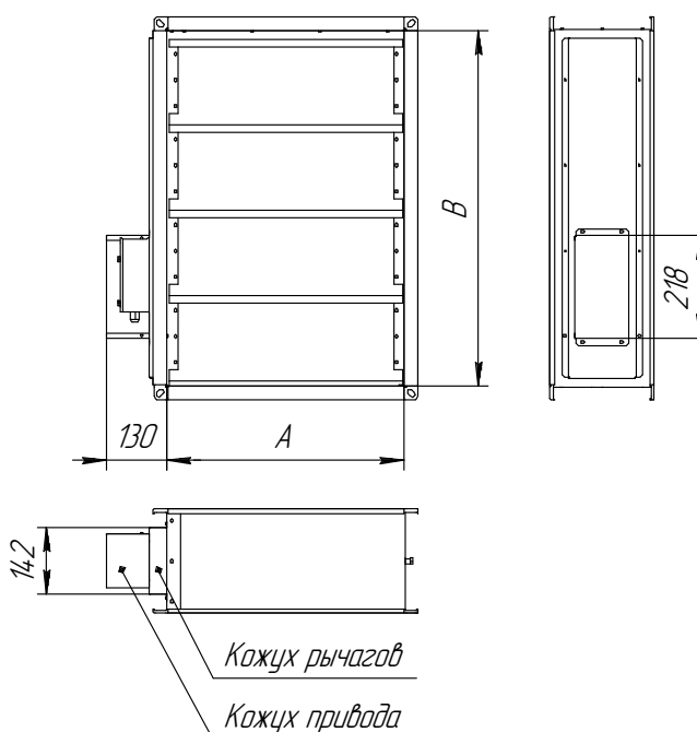
Клапан KPNZ-90-F2-SN-MN-ML, исполнение 04 с KZ
