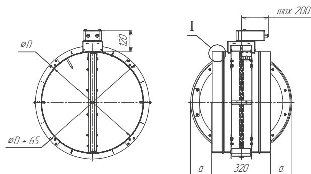
Рисунок 4 — Ниппельное исполнение 500 \leq D \leq 1000
