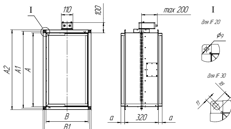
Рисунок 1 — Исполнение без кожуха
