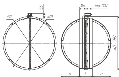
Рисунок 7 — Ниппельное исполнение D ≥ 1120
