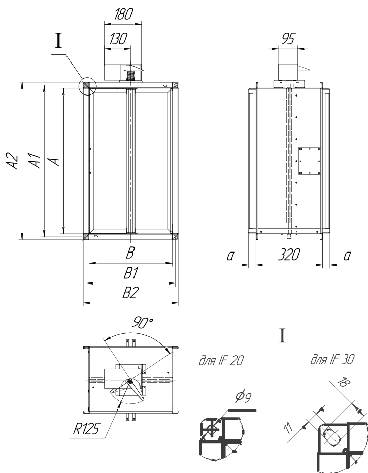
Рисунок 1 — Исполнение 04 с электромагнитным приводом
