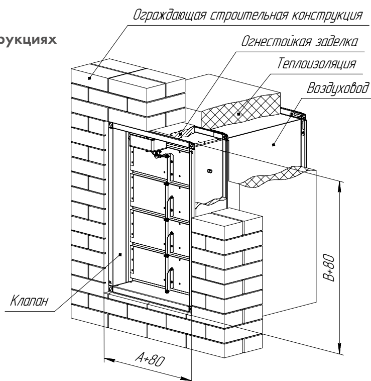
Клапан KD ML канальный с электромеханическим приводом внутри
