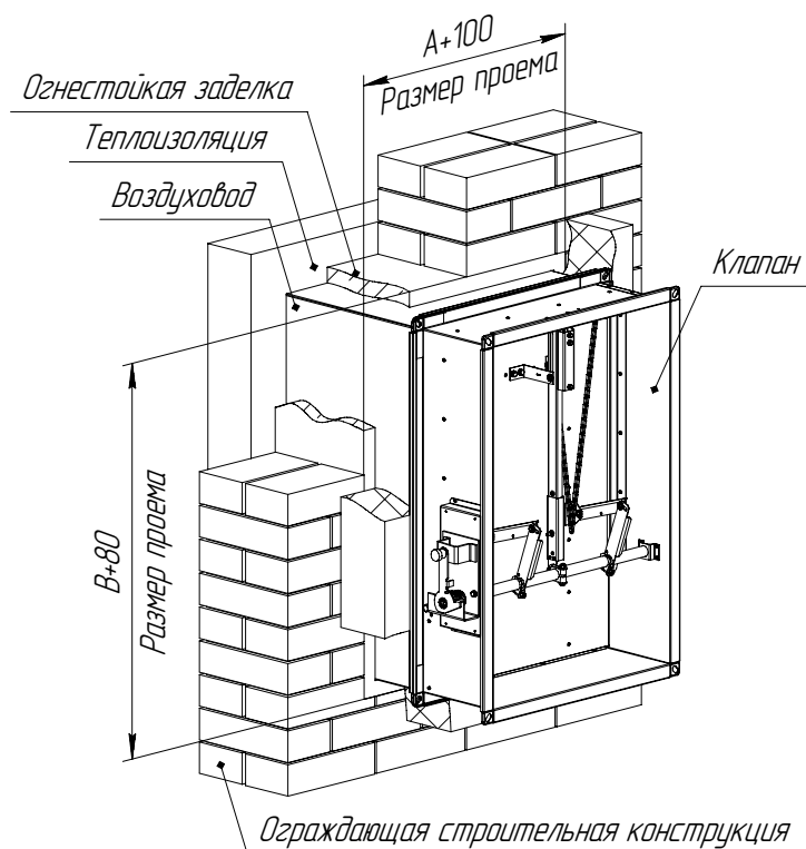
Клапан КД каналный с электромагнитным приводом снаружи
