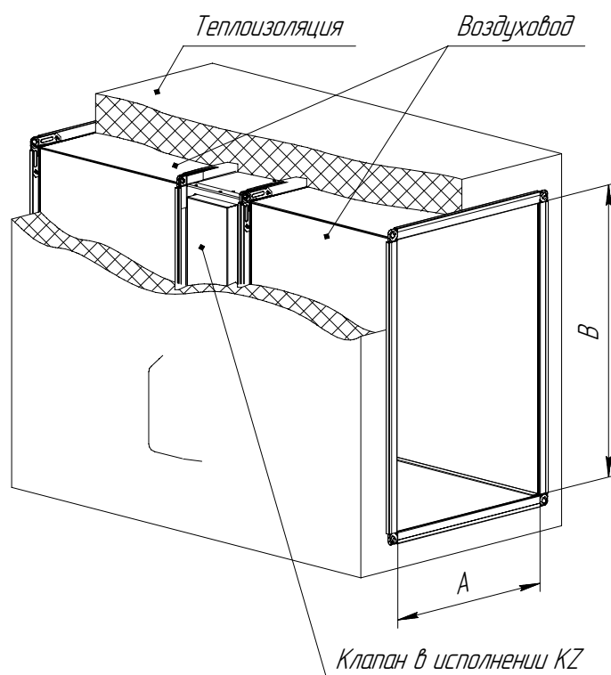
Клапаны KD ML и KD канальные с электромеханическим приводом снаружи
