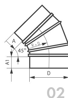
Отвод 45°
