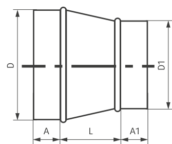
Переход центральный
