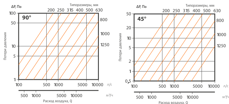
Отвод 90°
