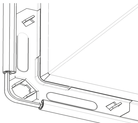
Интегрированный фланец TDC III с установленным уголком
