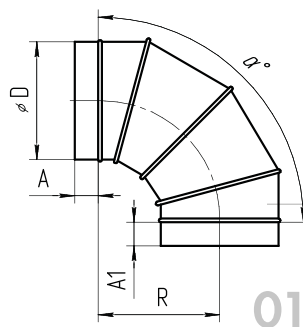
Отвод 90°
