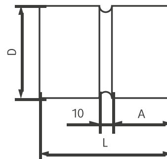
Ниппель наружный
