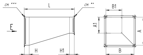
Вид Е
