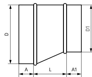
Переход односторонний
