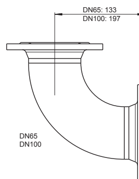
Размеры колен DN65 и DN100
