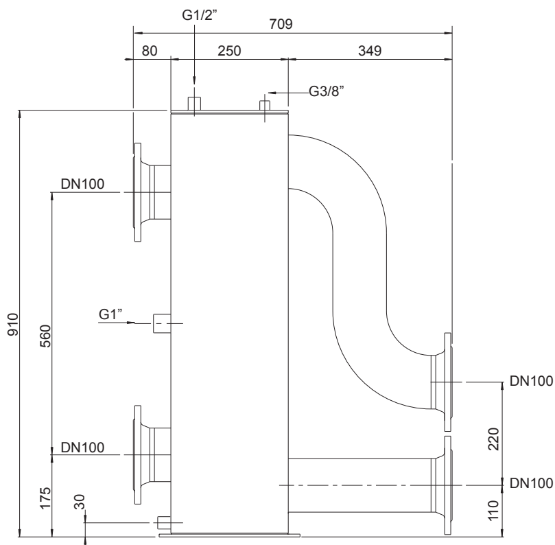
Размеры гидравлического разделителя DN100 до 1000 кВт
