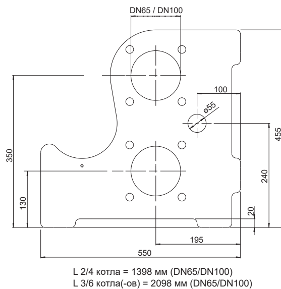
Размеры коллектора
