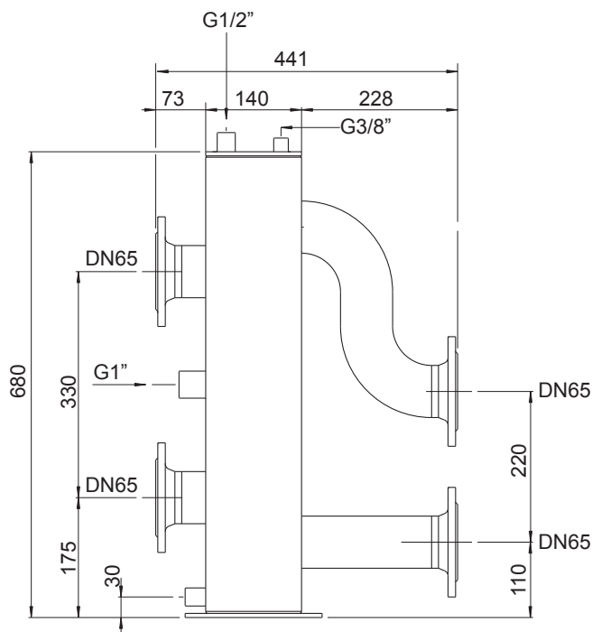
Размеры гидравлического разделителя DN65 до 452 кВт
