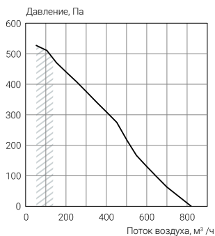
ECT PF-R 700
