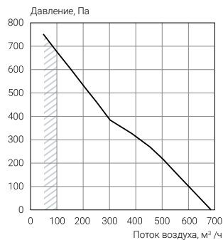
ECT PF-R 500
