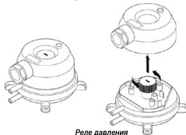
Реле давления
