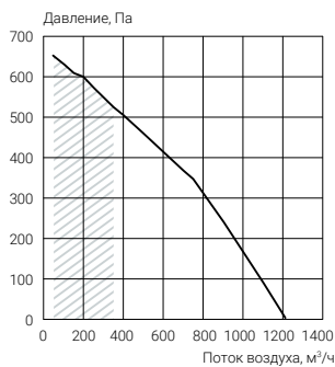
ECT PF-R 1150
