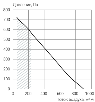
ECT PF-R 850
