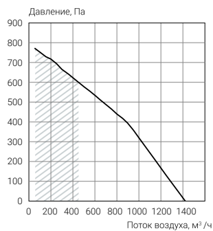
ECT PF-R 1350
