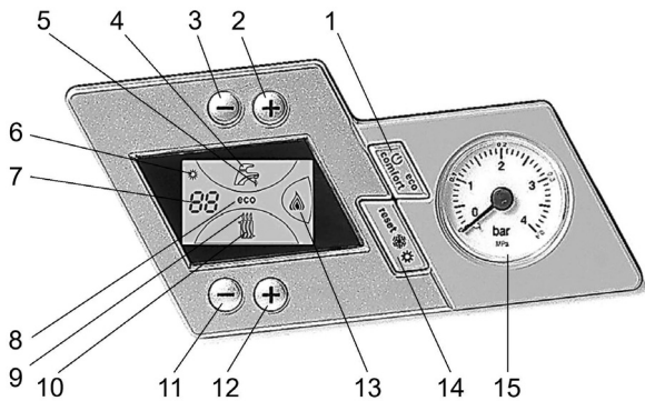
Рис. 1. Панель управления
