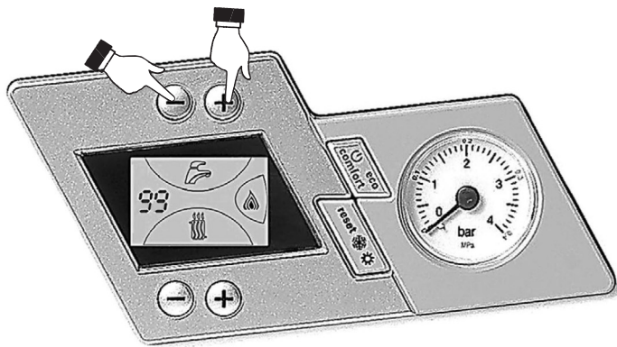
Рис. 13. Режим TEST (мощность системы отопления = 100%)
