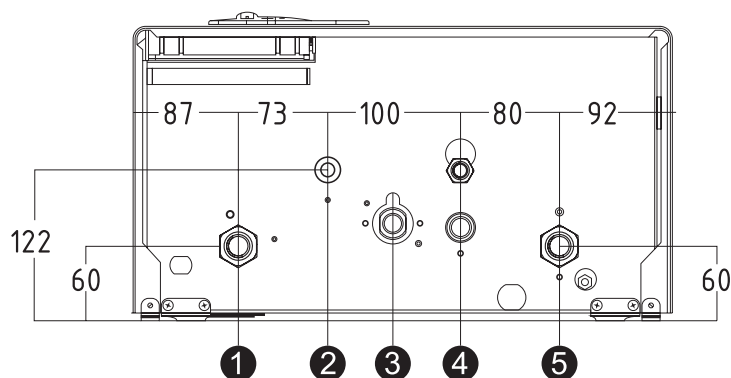
Рис. 4. Vitabel 10-24 кВт
