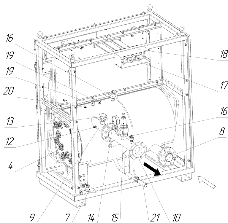
Рисунок 1 .Общий вид прибора (некоторые элементы условно не показаны)
