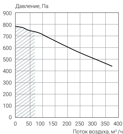
ECT PF-R 550-E1.0-R-4 Pro ECT PF-R 550-W-R-4 Pro
