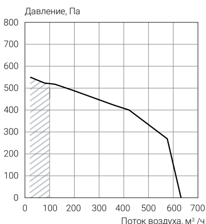
ECT PV-R 550-E1.0-(L/R)-4 Pro ECT PV-R 550-W-(L/R)-4 Pro
