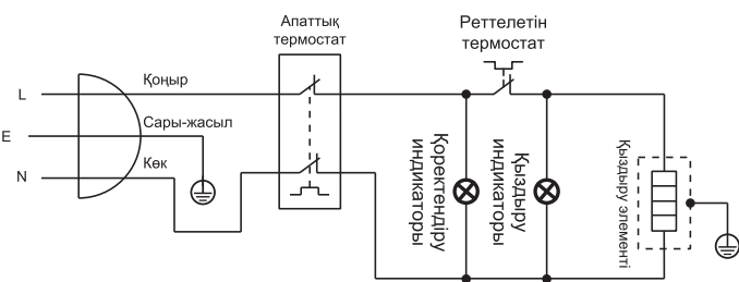
MQ1, MQ2 электр тізбегі
