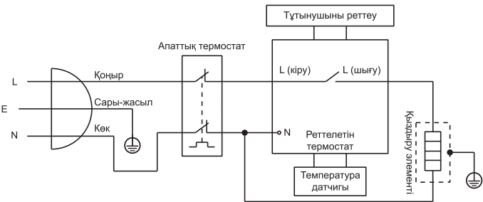
EQ1, EQ2 электр тізбегі
