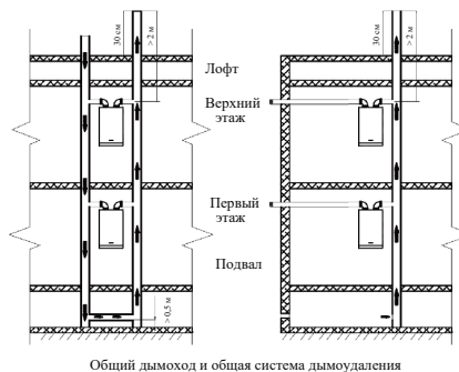
Общий дымоход и общая система дымоудаления
