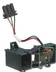
Контакт сигнализации электрического повреждения SDE1
