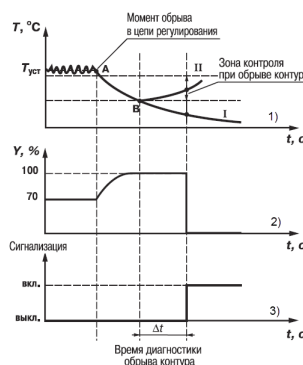
Рисунок 7.13 – Срабатывание LBA
