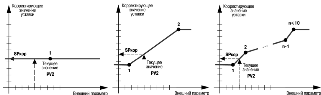
Рисунок 7.6 – График коррекции уставки
