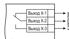
Рисунок 5.12 – Схема подключения нагрузки к ВУ типа Р
