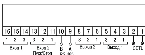
Рисунок 5.3 – Назначение контактов клеммника TPM212-H2
