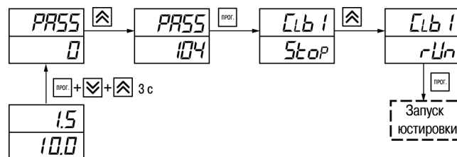
Рисунок 8.2 – Запуск юстировки
