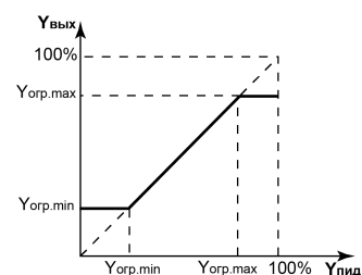
Рисунок 7.7 – Ограничение выходного сигнала
