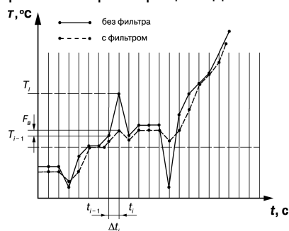
Рисунок 7.4 – Сглаживание единичных помех в зависимости от ширины полосы цифрового фильтра
