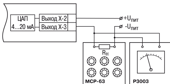
Рисунок 8.9 – Подключение ВУ1 типа У
