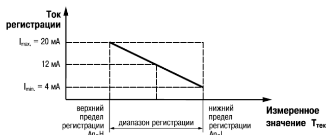
Рисунок 7.7 – Настройка при A_{n-L} > A_{n-H}
