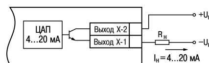
Рисунок 5.18 – Подключение к ВУ типа И
