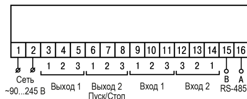
Рисунок 5.2 – Общая схема подключения TPM210-H, -Щ1 и -Щ2
