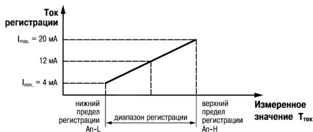
Рисунок 7.6 – Настройка при A_{n-L} < A_{n-H}
