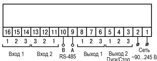
Рисунок 5.3 – Общая схема подключения TPM210-H2
