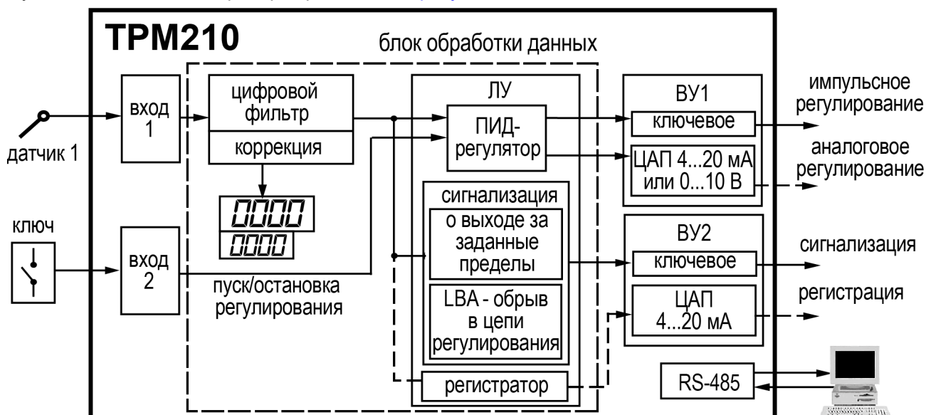
Рисунок 6.1 – Функциональная схема прибора
