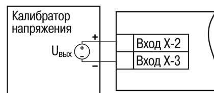
Рисунок 8.4 – Схема подключения при юстировке ТП
