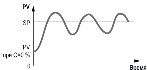
Рисунок 7.12 – Колебания в системе «нагреватель»
