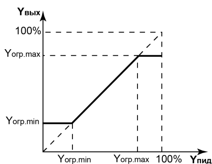
Рисунок 7.10 – Ограничение значения выходного сигнала
