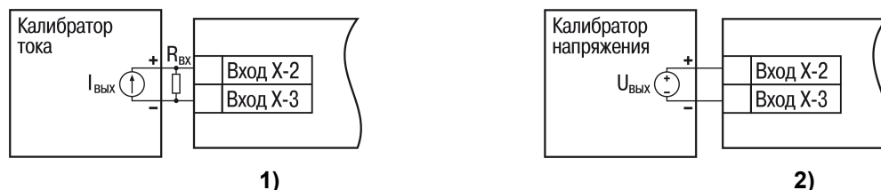
Рисунок 8.6 – 1) постоянный ток, 2) постоянное напряжение
