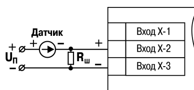
Рисунок 5.10 – Схема подключения пассивного датчика с токовым выходом 0...5 мА или 0 (4)...20 мА R_{ш} = 100 \pm 0,1 \text{ Ом}
