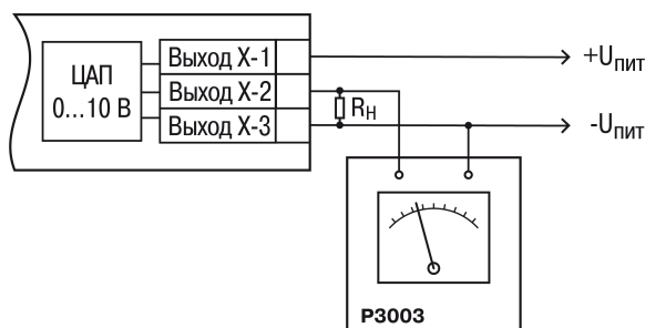
Рисунок 8.8 – Подключение ВУ1 типа И ( R_H = 500 \text{ Ом} )
