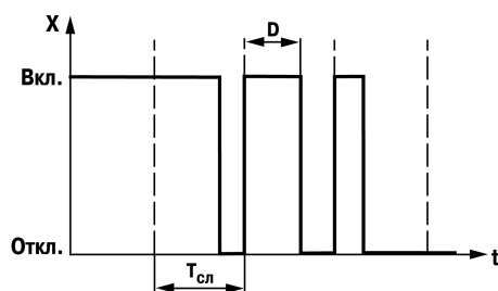
Рисунок 7.11 – Временная диаграмма выходного сигнала ПИД-регулятора
