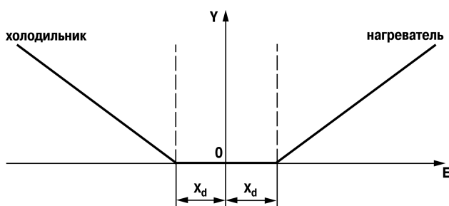
Рисунок 7.12 – Управление нагревателем и холодильником с зоной нечувствительности
