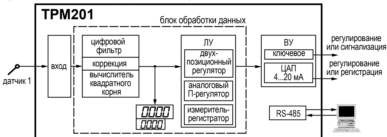
Рисунок 6.1 – Функциональная схема прибора
