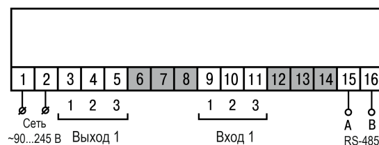
Рисунок 5.2 – Общая схема подключения TPM201-H, -Щ1 и -Щ2
