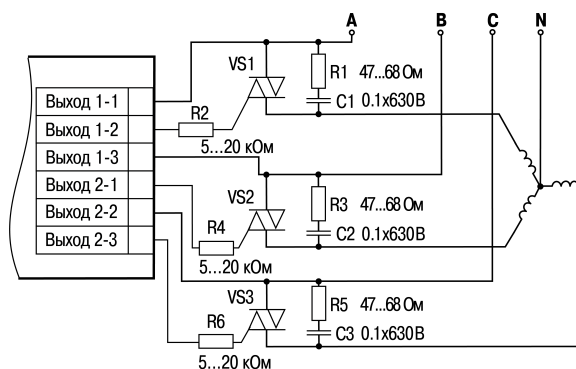
Рисунок 5.16 – Схема подключения силового симистора к ВУ типа С3
