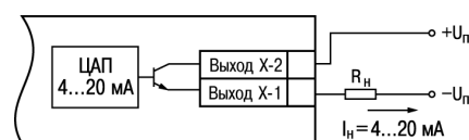
Рисунок 5.17 – Подключение к ВУ типа И
