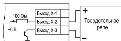
Рисунок 5.13 – Схема подключения нагрузки к ВУ типа Т
