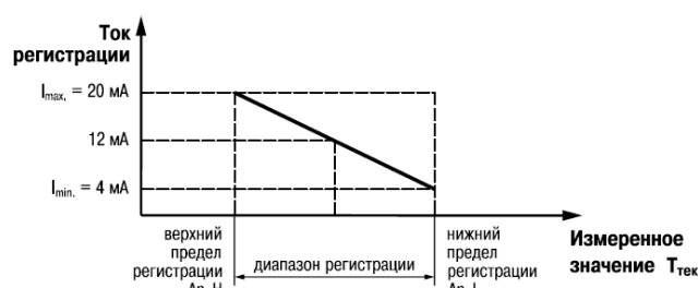
Рисунок 7.7 – Настройка диапазона в случае An.L > An.H
