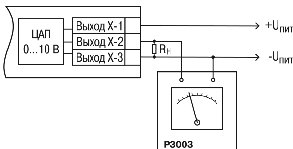
Рисунок 8.9 – Подключение ВУ1 типа У
