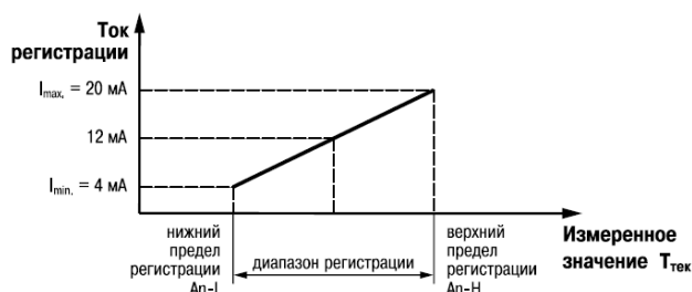
Рисунок 7.6 – Настройка диапазона в случае An.L < An.H
