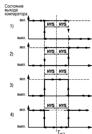
Рисунок 7.9 – Типы логики работы регулятора
