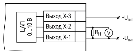
Рисунок 5.19 – Схема подключения нагрузки к ВУ типа У
