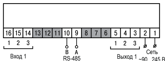
Рисунок 5.3 – Общая схема подключения TPM201-H2
