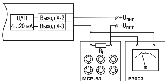
Рисунок 8.8 – Подключение ВУ1 типа И (R н =500 Ом)
