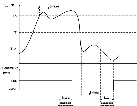
Рисунок 7.10 – Работа с задержками и удержанием
