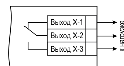
Рисунок 5.11 – Схема подключения нагрузки к ВУ типа Р
