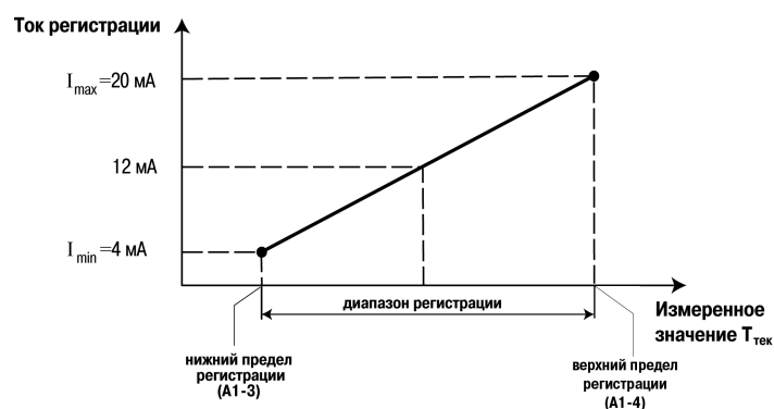
Рисунок 7.12 – Принцип формирования тока регистрации
