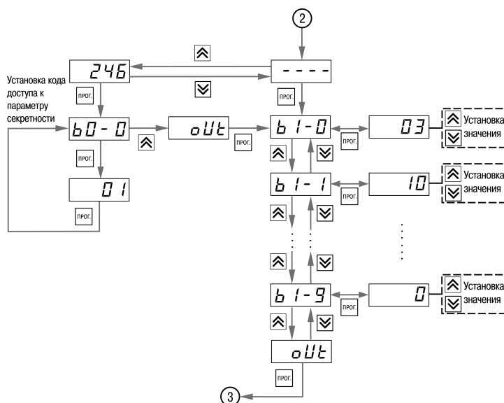
Рисунок 7.4 – Последовательность работы с прибором на втором уровне настройки (для группы параметров В)
