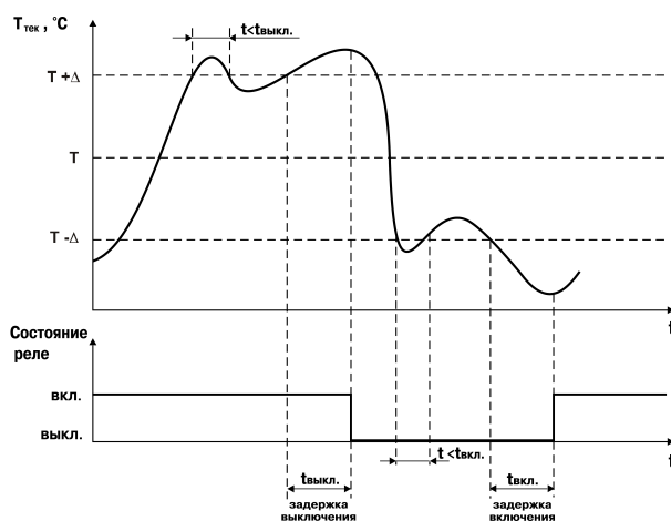
Рисунок 7.9 – Задание задержек включения/выключения ВУ для типа логики 1
