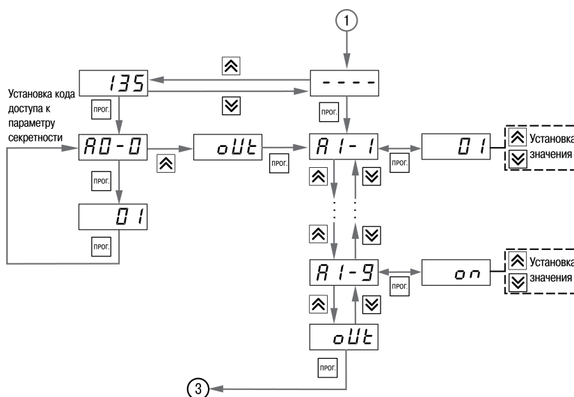
Рисунок 7.3 – Последовательность работы с прибором на втором уровне настройки (для группы параметров А)
