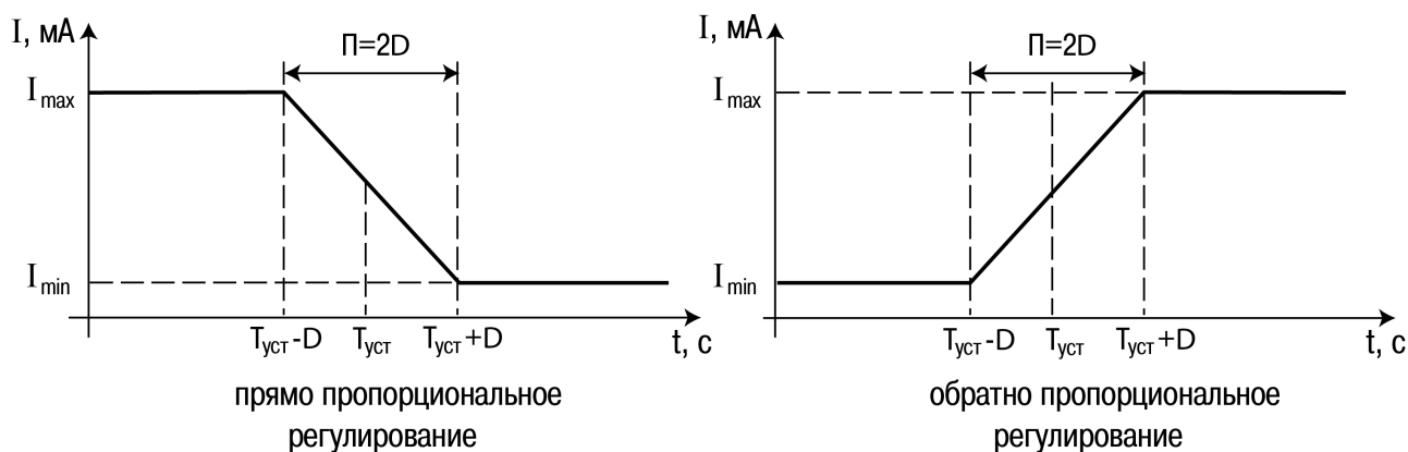
Рисунок 7.11 – Принцип формирования управляющего тока П-регулятора
