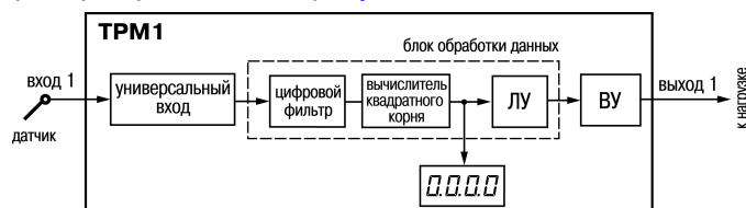
Рисунок 6.1 – Функциональная схема прибора
