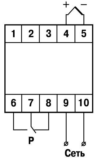
Рисунок 3 – Общая схема подключения
