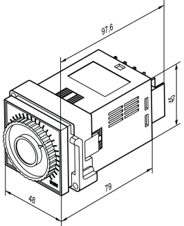
Рисунок 1 – Габаритные размеры
