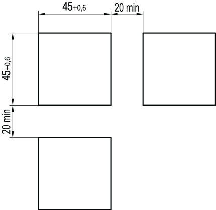
Рисунок 2 – Разметка отверстий в лицевой панели щита под крепление нескольких приборов
