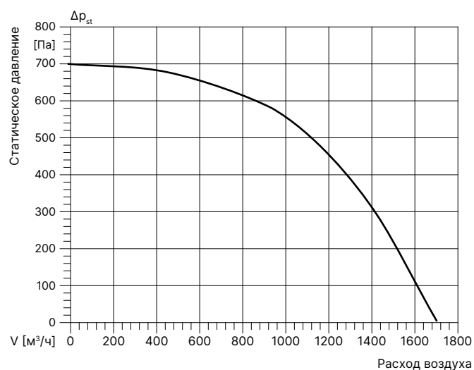
КВН-М (ШГ) 50-30/22-0,25-2D
