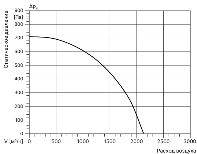
КВН-М (ШГ) 60-35/25-0,37-2D
