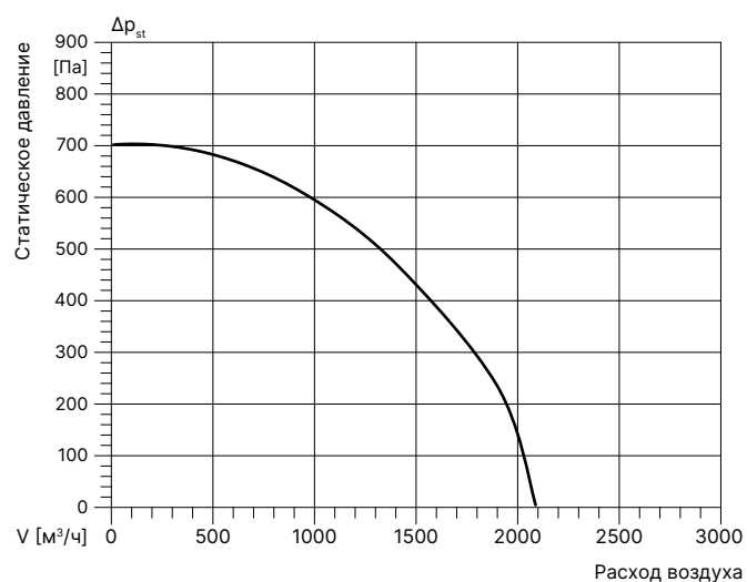
КВН-М (ШГ) 60-30/25-0,37-2D
