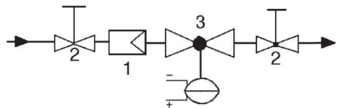
Обвязка регулятора перепада давления
