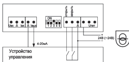
Схема подключения в режиме трехпозиционного управления (беспотенциальный контакт или открытый коллектор)
