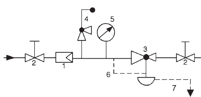
Обвязка перепускного клапана для жидкостей и газов
