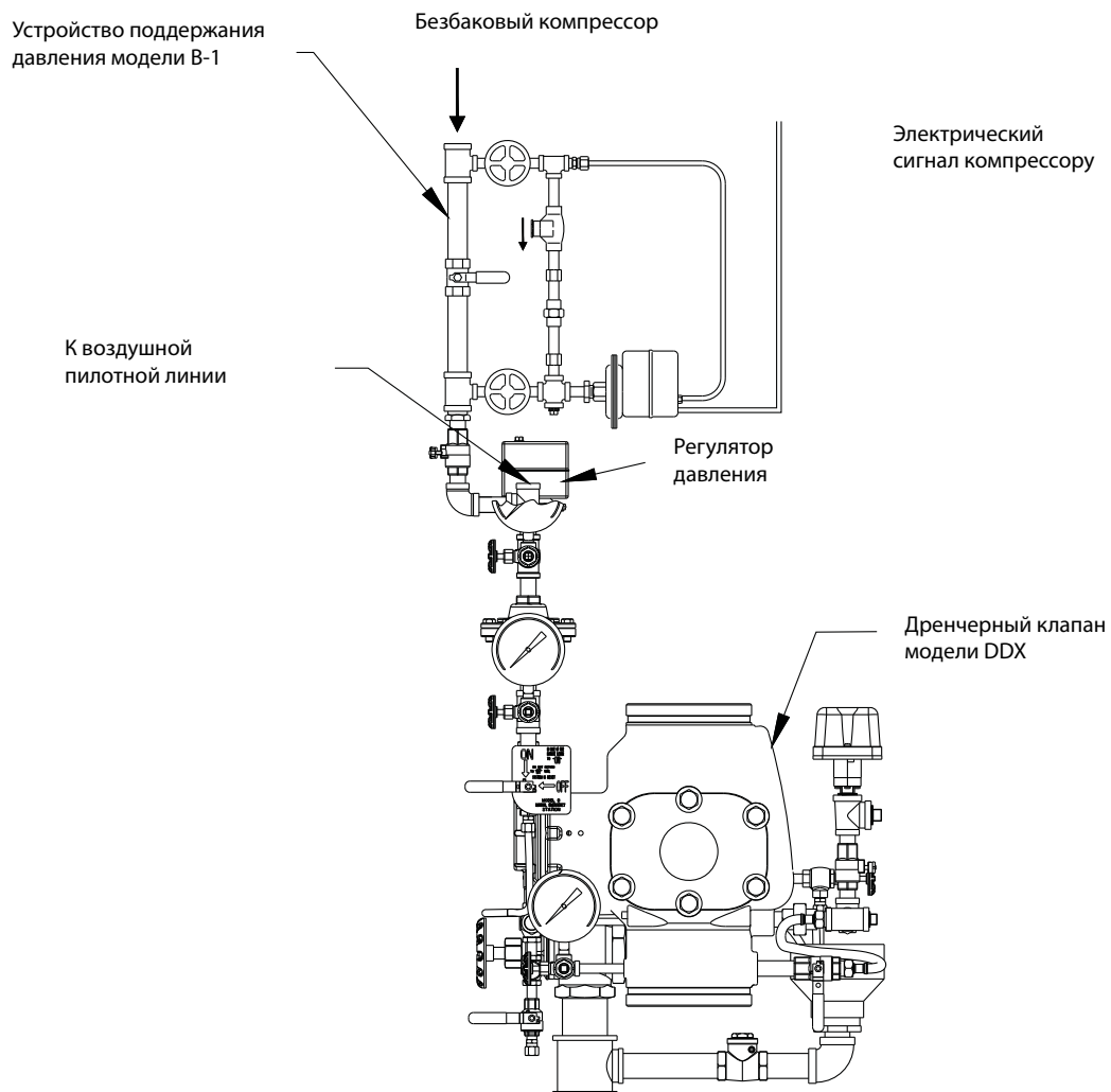
Схема установки модели В-1 с клапаном модели DDX (сухой пуск)
