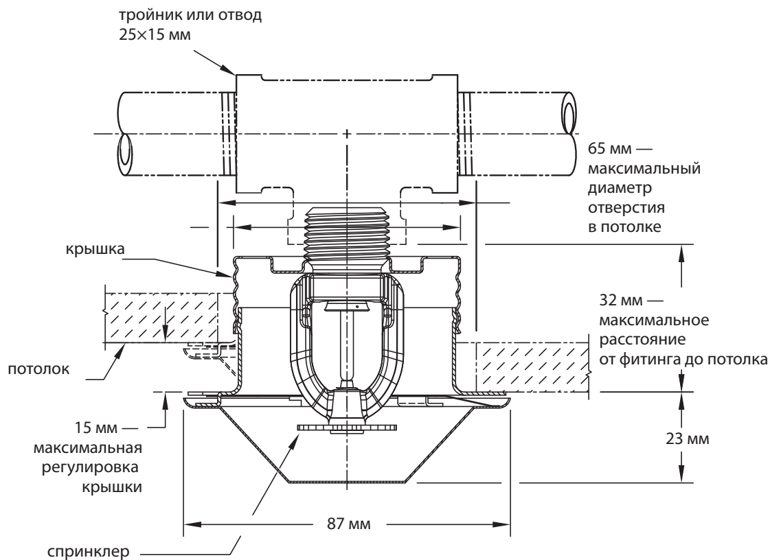
Схема монтажа оросителя RA1414
