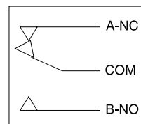
Рис. 6. Схема переключателя в состоянии «нет потока воды»
