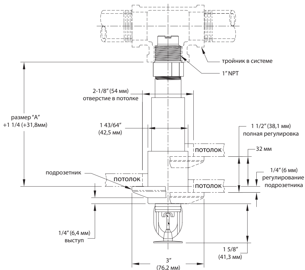
Схема монтажа оросителя R5714 со стандартным цоколем
