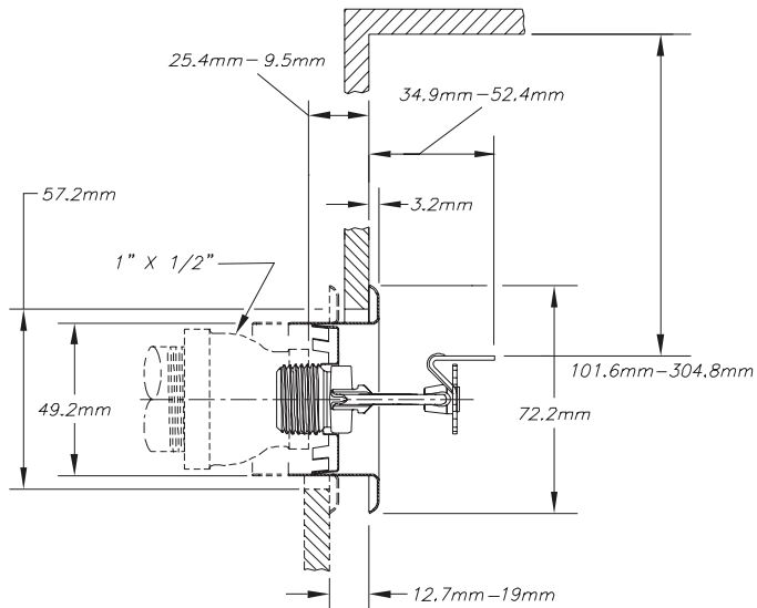
Схема монтажа оросителя RA1335, RA1435
