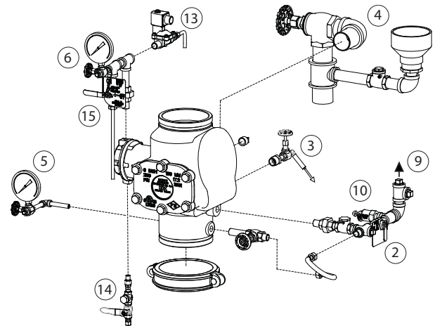
Клапан воздушный DDX с обвязкой для сухого пилотного пуска, соответствующей стандартам FM*
