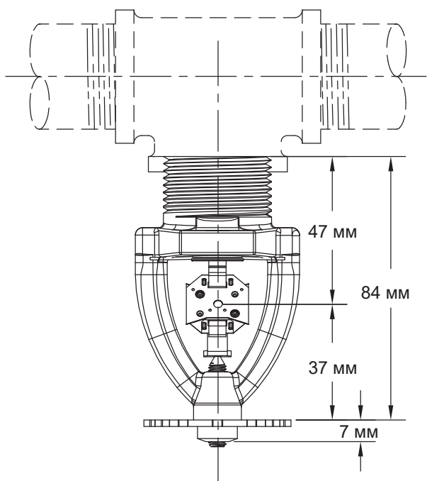
Схема монтажа оросителя RA0842
