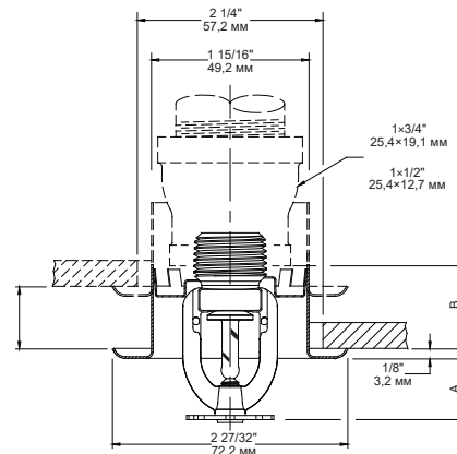
Схема монтажа оросителя с фасонным цоколем
