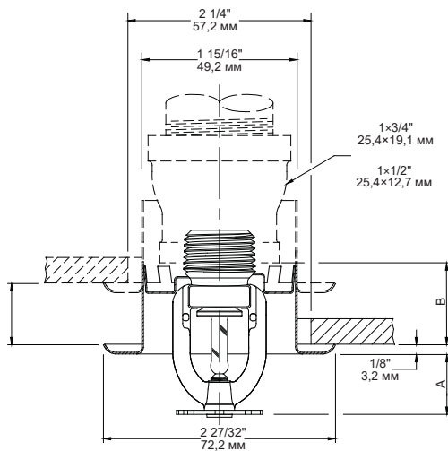
Схема монтажа оросителя RA2745 с фасонным цоколем
