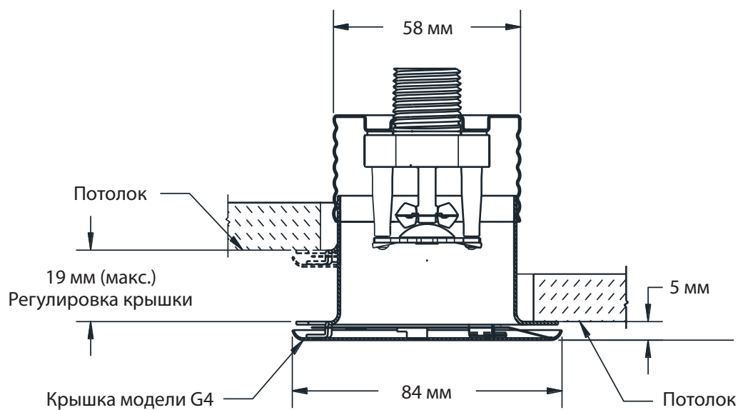
Схема монтажа оросителя RA3415
