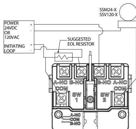
Рис. 5. Электрическая схема
