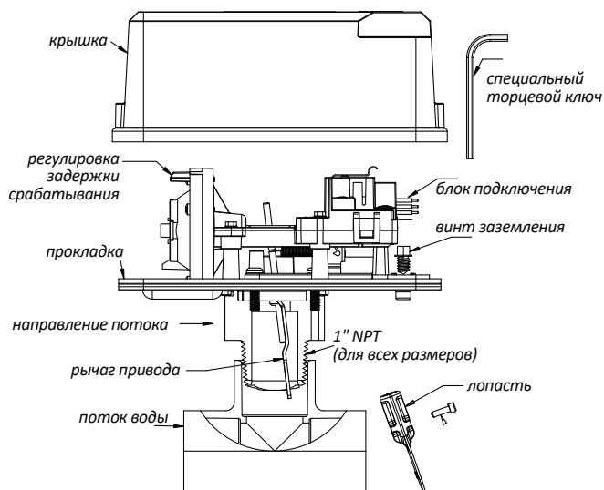
Рис. 2. Схема установки модели WFDN
