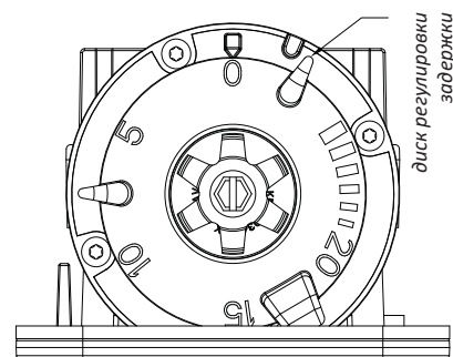
Рис. 4. Шкала регулировки времени задержки срабатывания
