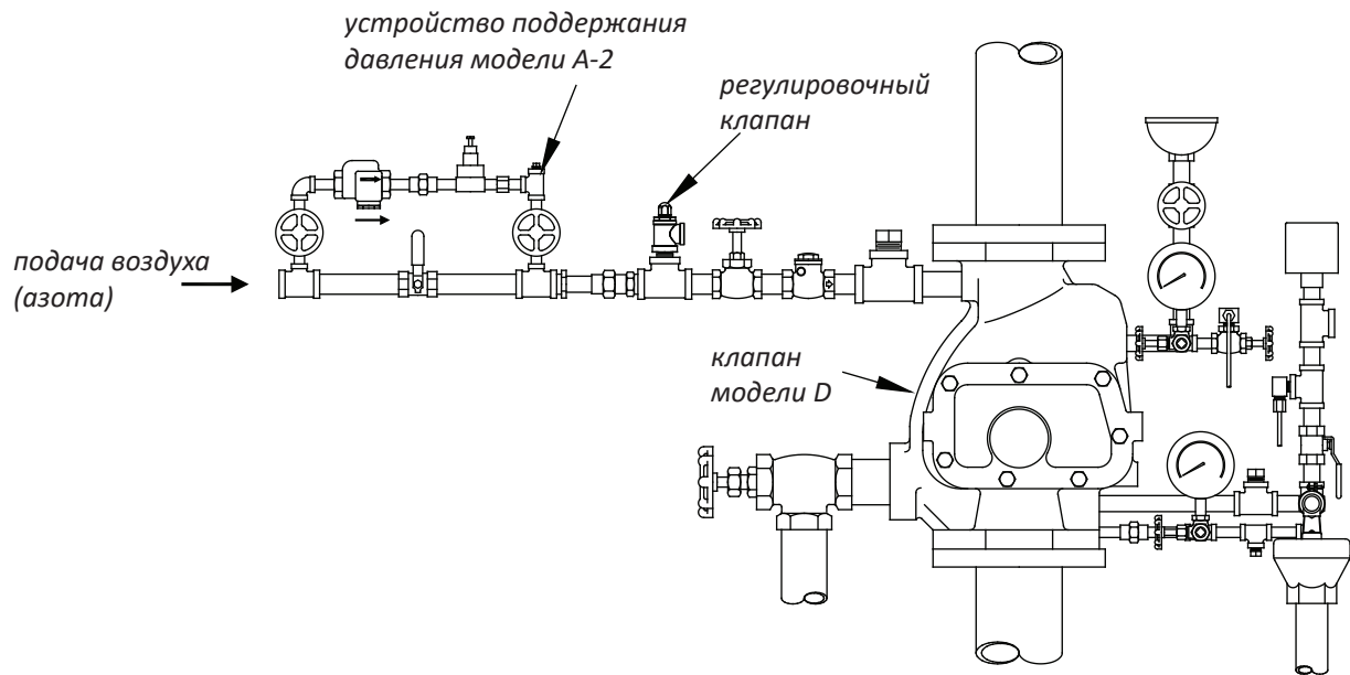
Схема установки устройства поддержания давления модели A2 с воздушным клапаном модели D
