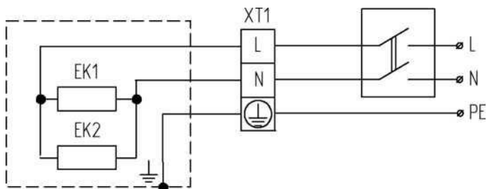
Рис. 1 Обогреватель для TIR-EP-P0.6-54, TIR- EP-P0.8-54, TIR- EP-P1.0-54
