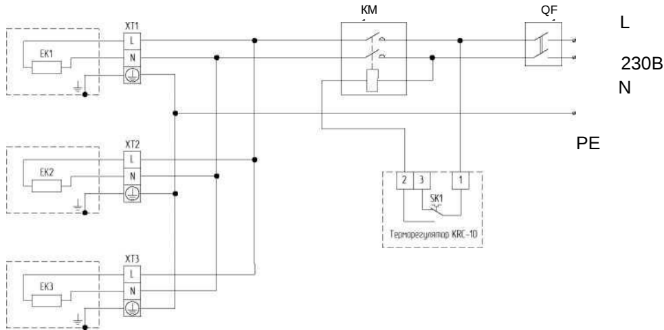
Рис. 1 Обогреватель для TVI- EP-P0.6-54, TVI-EP-P0.8-54, TVI- EP-P1.0-54
