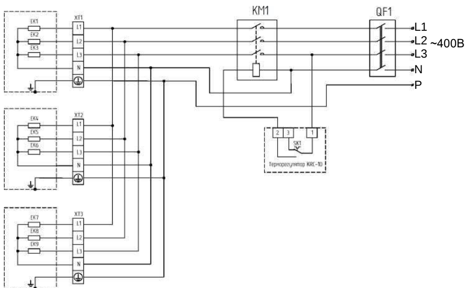
Рис. 3 Обогреватель для TVI-EP-P3.0-54, TVI-EP-P4.0-54
