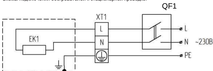
Рис. 1 Обогреватель для TIR-EP-P0.6-54, TIR- EP-P0.8-54, TIR- EP-P1.0-54
