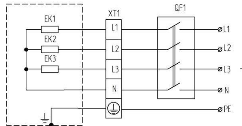
Рис. 3 Обогреватель для TIR- EP-P3.0-54, TIR- EP-P4.0-54
