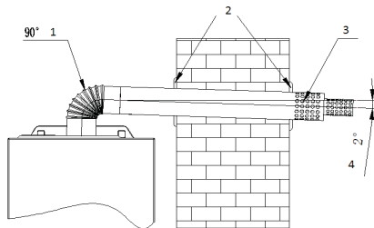
1- 90° патрубок; 2-фланец трубы дымоотвода; 3- труба дымоотвода; 4-уклон 2°
