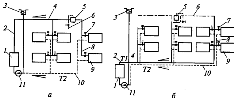
Рис. 3.3. Двухтрубные системы водяного отопления с принудительным побуждением:
