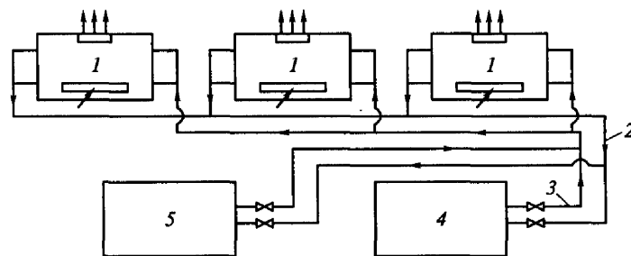
Рис. 9.13. Схема системы местного кондиционирования:
