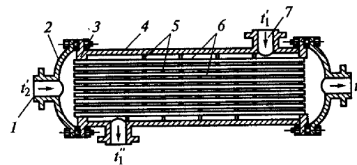
Рис. 1.6. Водоводяной подогреватель:
