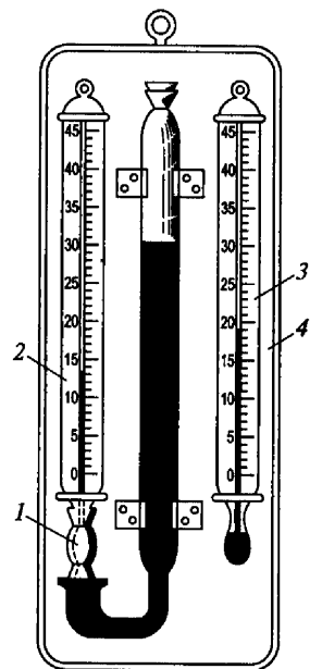
Рис. 10.6. Психрометр:
