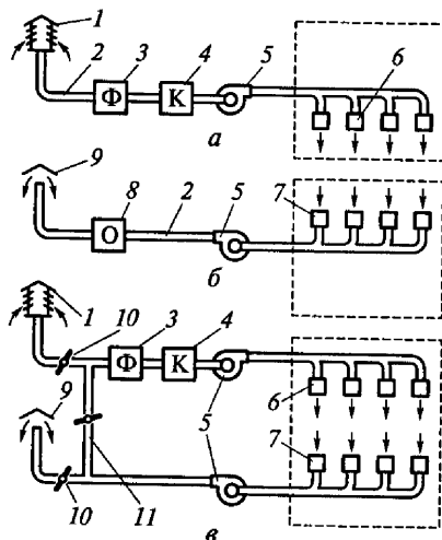
Рис. 7.2. Схемы механической вентиляции:
