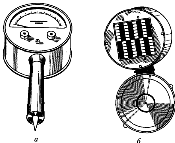
Рис. 10.10. Актинометр:
