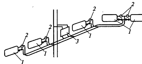
Рис. 5.7. Система отопления с горизонтальными двухконтурными ветками для параллельно-последовательно подсоединенных отопительных приборов: 1 — отопительные приборы; 2 — встроенные терморегуляторы; 3 — квартирный тепловой пункт
