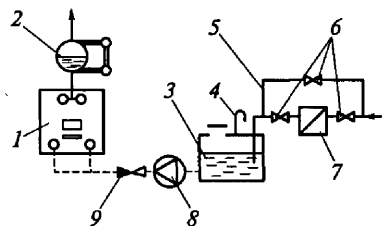
Рис. 3.17. Схема принудительного возврата конденсата:
