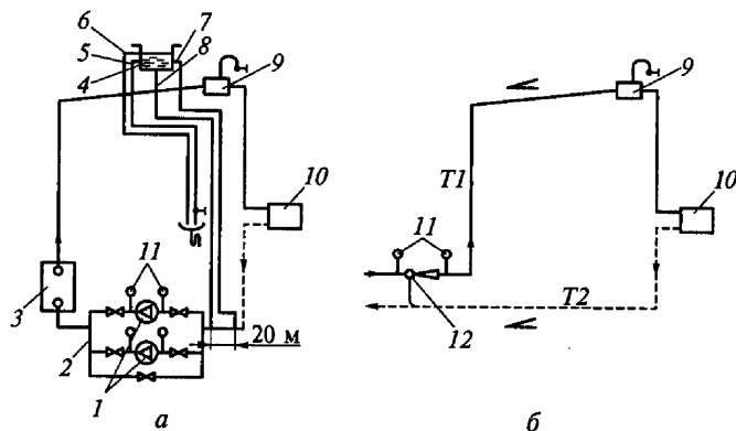
Рис. 3.10. Системы водяного отопления с принудительным побуждением: а — от насоса; б — с помощью водоструйного элеватора; 1 — циркуляционные насосы; 2 — обводная линия; 3 — котел; 4 — расширительный бак; 5 — контрольная труба; 6 — переливная труба; 7 — циркуляционная труба; 8 — расширительная труба; 9 — воздухоотборник; 10 — отопительный прибор; 11 — манометры; 12 — водоструйный элеватор
