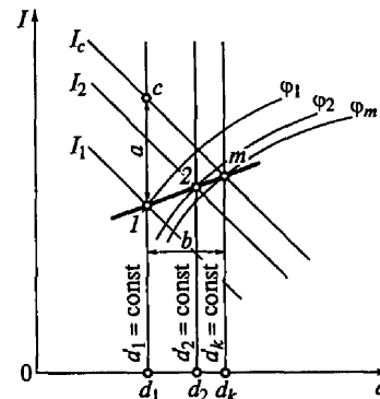
Рис. 6.4. Построение на I-d -диаграмме луча процесса изменения состояния воздушно-паровой смеси при добавлении в нее водяного пара
