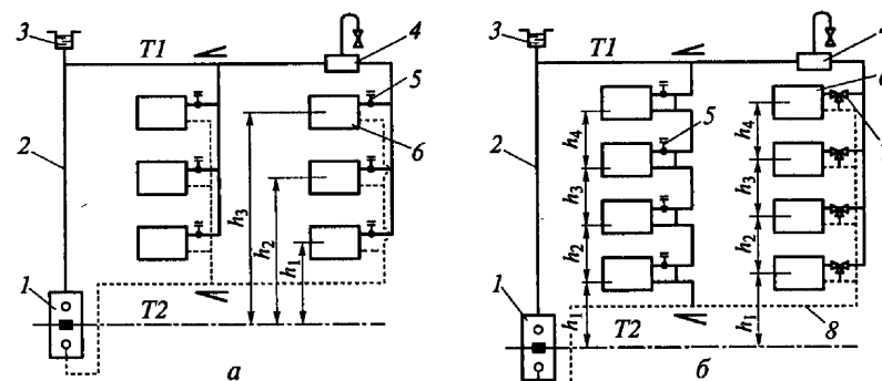
Рис. 3.8. Системы водяного отопления с естественным побуждением: а — двухтрубная; б — однотрубная; 1 — котел; 2 — главный стояк; 3 — расширительный бак; 4 — воздушник; 5 — кран двойной регулировки; 6 — отопительный прибор; 7 — трехходовой регулировочный кран; 8 — обратная магистраль
