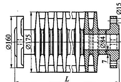
Рис. 4.4. Ребристая чугунная труба
