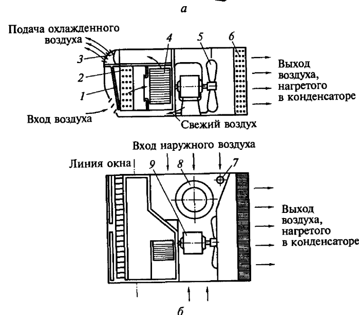
Рис. 9.14. Оконный кондиционер со встроенной холодильной машиной: а — общий вид; б — компоновка оборудования; 1 — фильтр; 2 — испаритель; 3 — регулирующие жалюзи; 4 — центробежный вентилятор; 5 — осевой вентилятор; 6 — конденсатор; 7 — фильтр-осушитель; 8 — компрессор; 9 — электродвигатель
