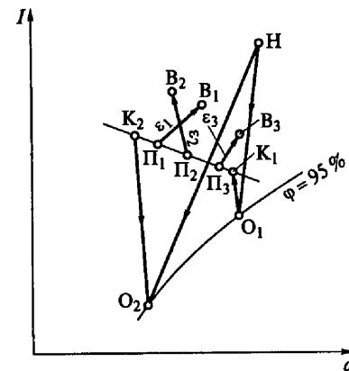
Рис. 9.12. Построение на I-d -диаграмме процесса кондиционирования при применении двухканальной системы подачи приточного воздуха
