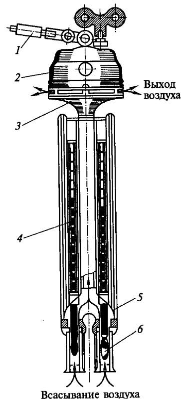
Рис. 10.7. Аспирационный психрометр с вентилятором:
