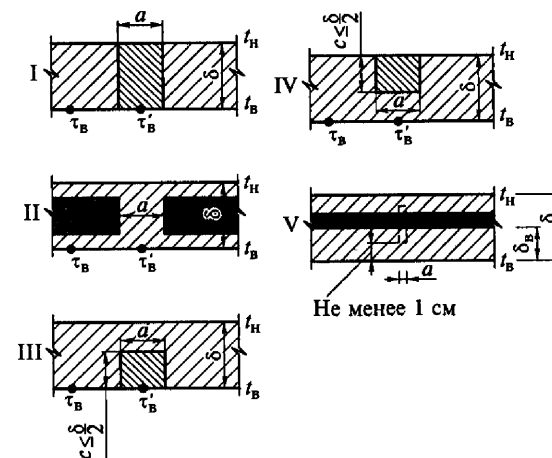
Рис. 2.3. Варианты схем теплопроводных включений в ограждающие конструкции
