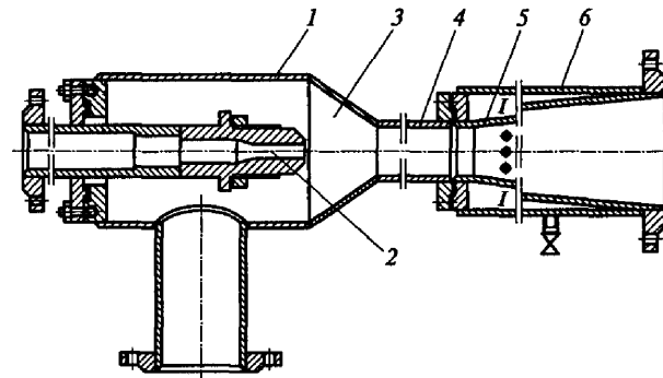
Рис. 11.6. Паровой инжектор:
