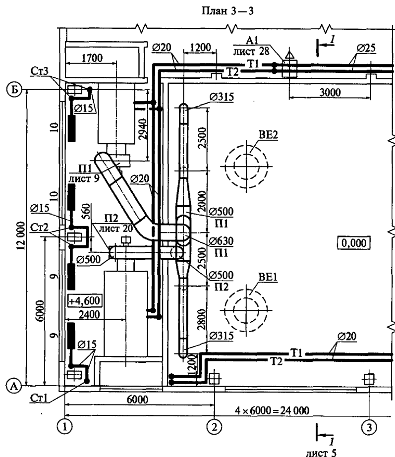
Рис. 12.1. Чертеж части плана производственного здания с сетями отопления и вентиляции
