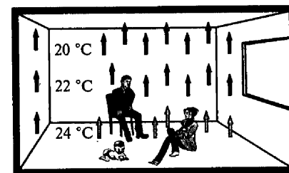
Рис. 3.29. Схема тепловых потоков в помещении с подогреваемым полом
