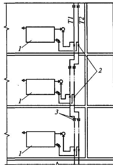
Рис. 4.8. Схема присоединения отопительных приборов к стоякам отопления из металлополимерных труб:
