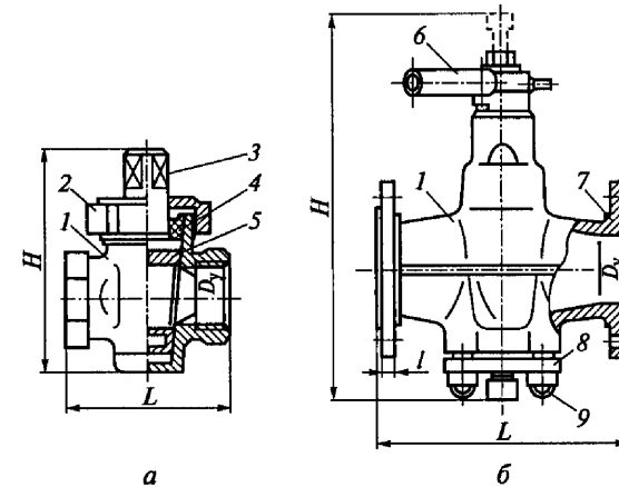
Рис. 5.3. Пробковые краны:
