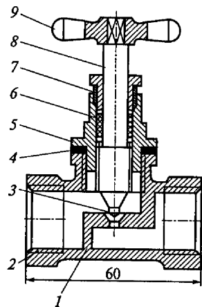
Рис. 5.4. Дроссельный регулирующий кран:
