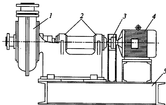
Рис. 3.11. Циркуляционный насосный агрегат:
