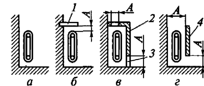
Рис. 4.9. Варианты установки отопительных приборов:
