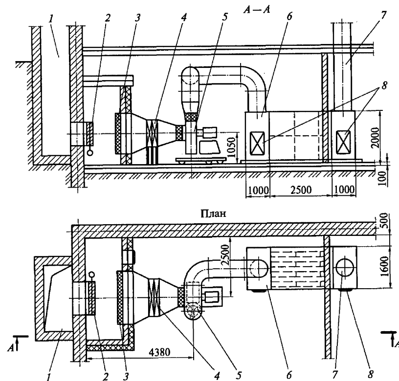
Рис. 8.10. Общий вид приточной вентиляционной камеры и размещенного в ней оборудования:
