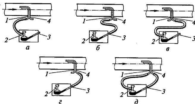
Рис. 10.4. Схемы присоединения пневмометрической трубки к напоромеру при замерах давления:
