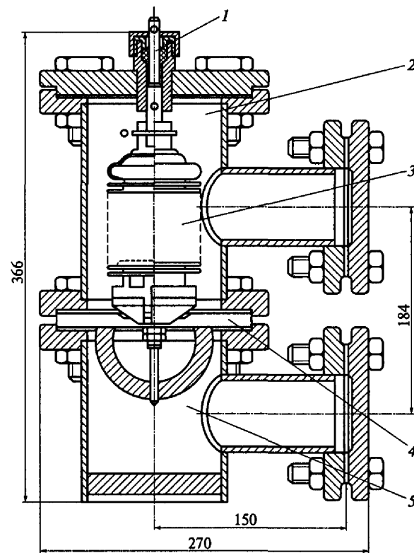
Рис. 11.7. Регулирующий клапан в сборе:
