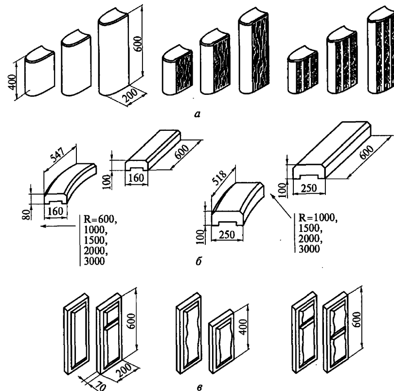
Рис. 2.2. Изделия из архитектурного бетона:
