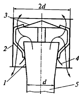
Рис. 7.7. Дефлектор ЦАГИ:
