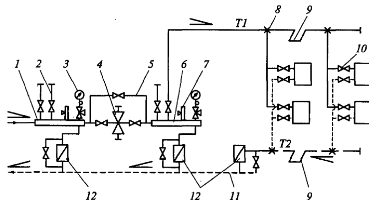
Рис. 3.19. Схема парового отопления высокого давления:
