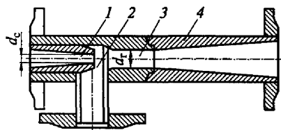
Рис. 3.13. Водоструйный элеватор: 1 — сопло; 2 — обратная труба; 3 — смеситель; 4 — диффузор
