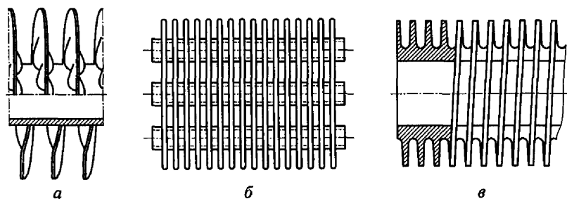
Рис. 8.5. Виды оребрения калориферов:
