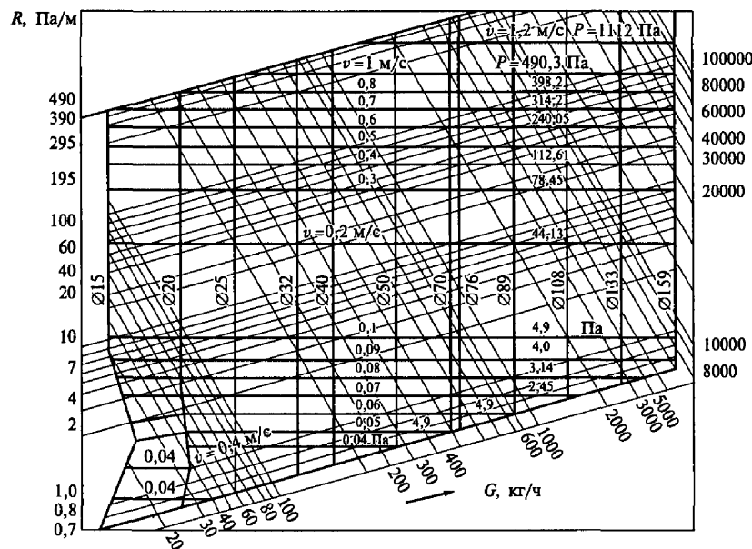
Рис. 3.15. Номограмма для расчета диаметров трубопроводов систем отопления при температуре воды 95...70 °С
