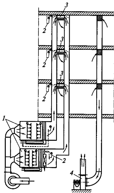
Рис. 9.11. Двухканальная система кондиционирования воздуха: 1 — кондиционеры; 2 — термостаты; 3 — смесители; 4 — вытяжной вентилятор
