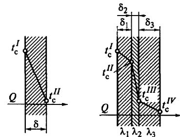
Рис. 1.3. Передача теплоты через плоскую стенку:
