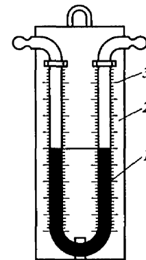
Рис. 10.1. U-образный манометр:
