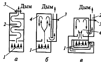
Рис. 3.24. Схемы дымоходов отопительных печей:
