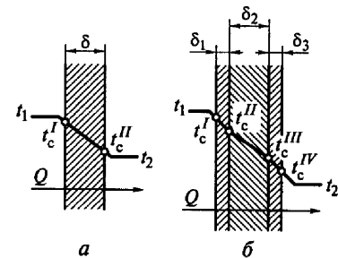
Рис. 1.4. Передача теплоты от греющей жидкости нагреваемой среде через разделительную стенку: а — однослойную; б — многослойную
