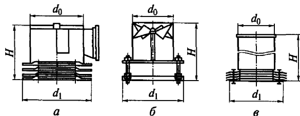
Рис. 8.6. Общий вид воздухораспределителей типа ВЭЦ (а), ВЭПв (б) и ВЭП (в)
