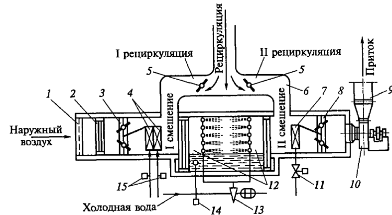
Рис. 9.1. Схема форсуночного кондиционера с I и II регулируемыми рециркуляциями:
