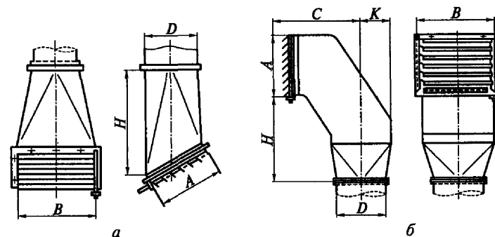
Рис. 8.7. Общий вид душирующих патрубков типа ПДв (а) и ПДн (б)
