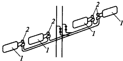
Рис. 5.8. Система отопления с горизонтальными однотрубными ветками для последовательно соединенных отопительных приборов: 1 — отопительные приборы; 2 — встроенные терморегуляторы
