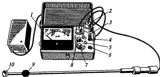
Рис. 10.5. Термоанемометр:
