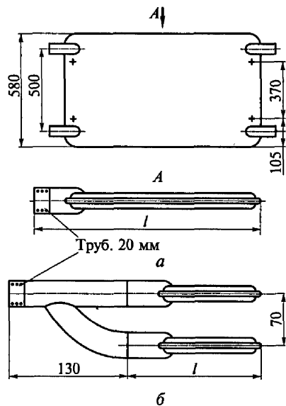
Рис. 4.3. Стальные панельные штампованные радиаторы типа РСВ: а — РСВ1-1; б — РСВ1-2
