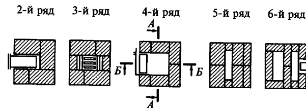
Рис. 3.25. Конструкция тонкостенной печи MBMC-61:
