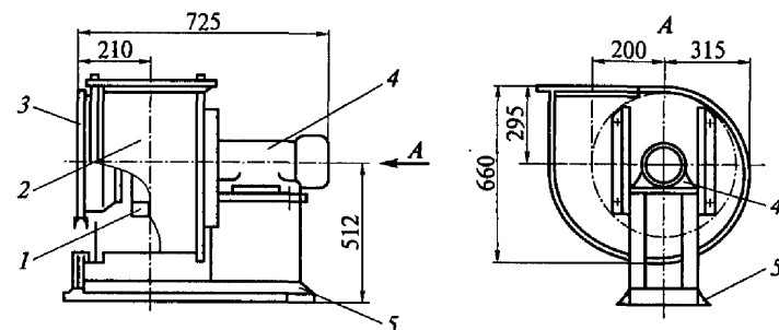
Рис. 8.2. Общий вид радиального (центробежного) вентилятора типа ВЦ4-70 № 4:
