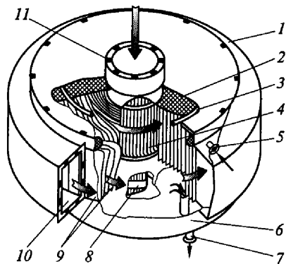
Рис. 11.2. Спиральный пленочно-контактный вентиляционный агрегат АСК-10:
