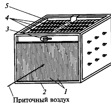
Рис. 11.4. Пленочно-контактная кассета для обработки приточного вентиляционного воздуха:
