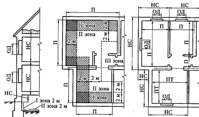
Рис. 3.1. Примеры обмера наружных ограждающих конструкций и пола здания:
