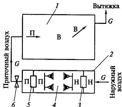
Рис. 9.2. Схема системы кондиционирования воздуха в летнее время с использованием адиабатического процесса обработки воздуха:
