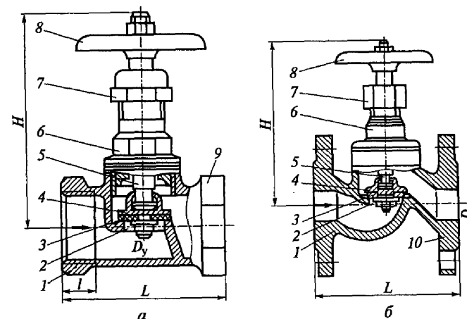
Рис. 5.2. Вентили:
