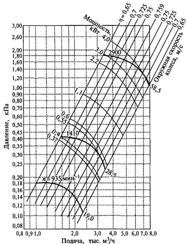
Рис. 8.3. Аэродинамическая характеристика вентилятора ВЦ4-70 № 4
