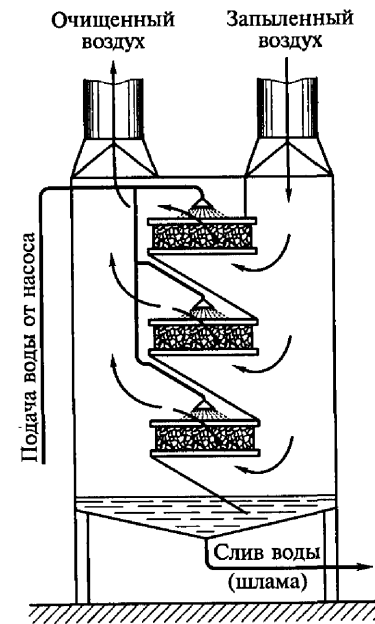
Рис. 8.9. Общий вид орошаемого фильтра
