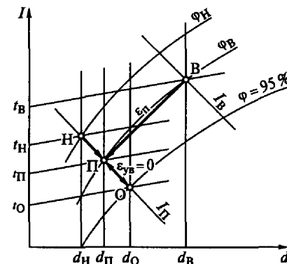
Рис. 9.5. Построение на I-d -диаграмме адиабатического процесса обработки воздуха в летнее время с подмешиванием части наружного воздуха в зоне за оросительной камерой
