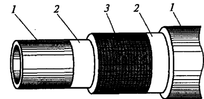
Рис. 5.6. Конструкция металлополимерной трубы:
