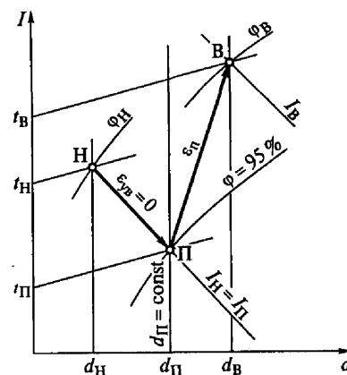
Рис. 9.3. Построение на I-d -диаграмме адиабатического процесса обработки воздуха в форсуночном кондиционере в летнее время
