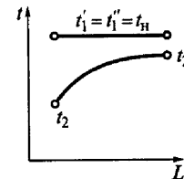
Рис. 1.9. График изменения температур греющего и нагреваемого теплоносителей по ходу (по длине L ) теплообменного аппарата, когда греющий теплоноситель — насыщенный пар
