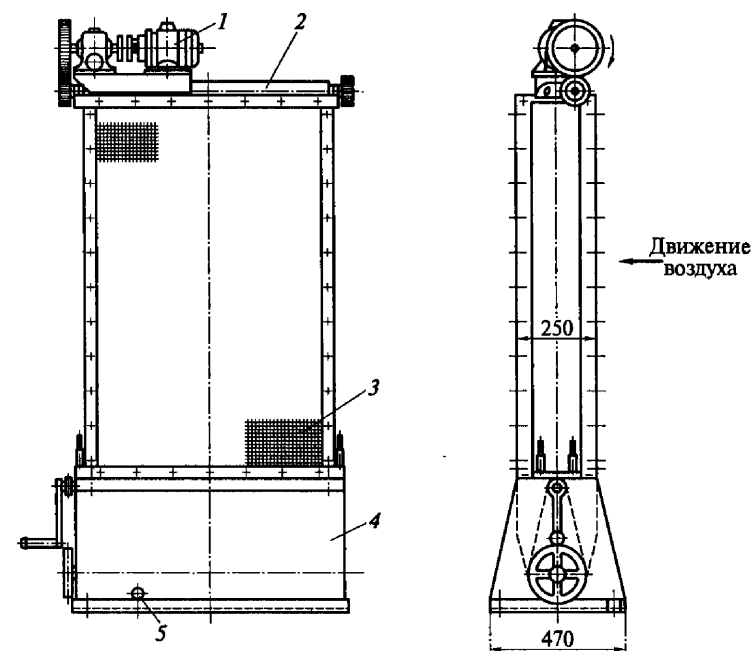
Рис. 9.9. Масляный самоочищающийся фильтр для очистки воздуха от пыли: 1 — электродвигатель; 2 — валик; 3 — сетка; 4 — масляная ванна; 5 — муфтовый кран
