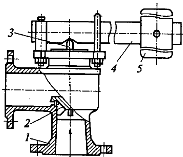
Рис. 5.5. Фланцевый предохранительный рычажно-грузовой клапан:
