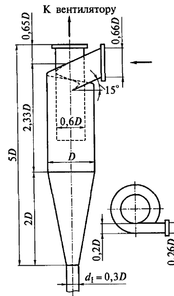
Рис. 8.8. Общий вид циклона
