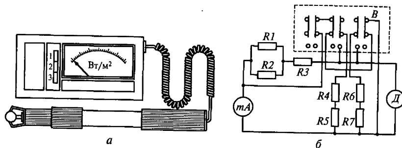
Рис. 10.9. Измеритель тепловых потерь ИТП-6:
