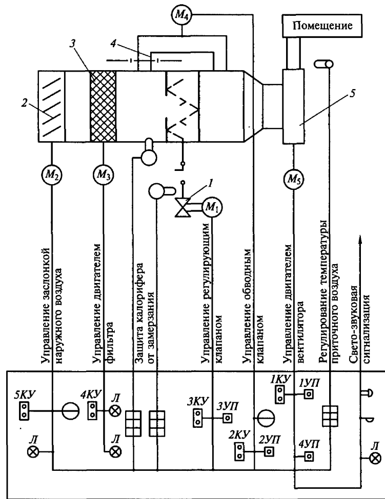
Рис. 11.8. Принципиальная схема автоматического управления вентиляционной системой:
