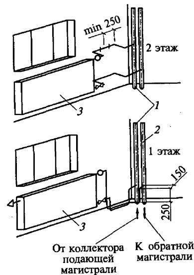
Рис. 3.2. Подсоединение отопительных приборов к стоякам из стальных труб:
