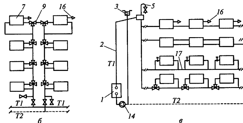
Рис. 3.4. Однотрубные системы водяного отопления с принудительным побуждением:
