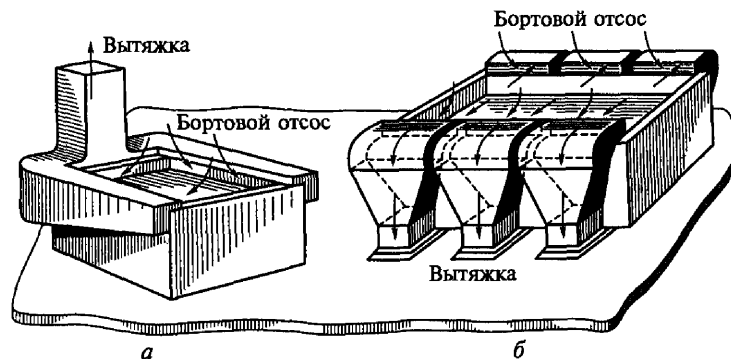
Рис. 7.10. Бортовые отсосы ванн:
