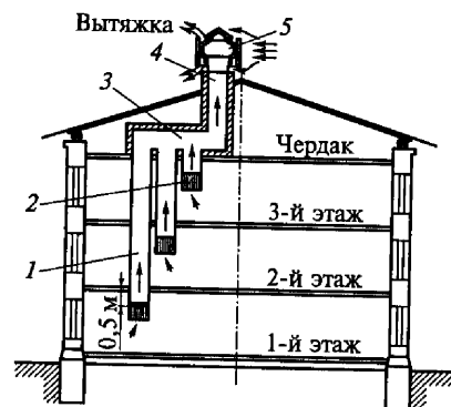
Рис. 7.6. Канальная система вытяжной вентиляции с естественным побуждением:
