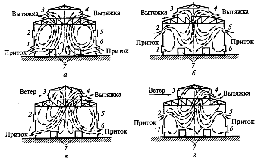
Рис. 7.5. Регулирование воздушных потоков при естественной вентиляции путем открывания створок:
