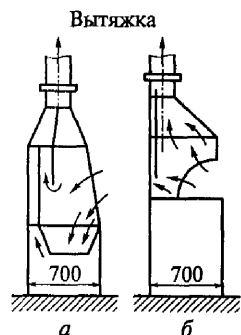
Рис. 7.9. Вытяжной шкаф: а — с нижним отсосом; б — с верхним отсосом
