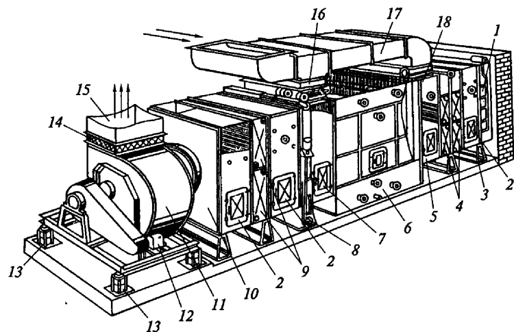
Рис. 9.6. Общий вид центрального форсуночного кондиционера типа КТЦ: 1 — приемный клапан; 2 — секции обслуживания; 3 — подставка; 4 — калориферы первого подогрева; 5, 7 — смесительные секции; 6 — камера орошения; 8 — секция воздушного фильтра; 9 — калориферы второго подогрева; 10 — переходная секция к вентилятору; 11 — вентиляционный агрегат; 12 — электродвигатель; 13 — виброамортизаторы; 14 — гибкая вставка; 15 — воздуховод приточного воздуха; 16 — рециркуляционный воздуховод; 17 — воздуховод первой рециркуляции воздуха; 18 — проходной клапан
