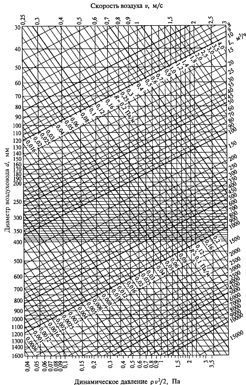
Рис. 7.8. Номограмма для расчета круглых стальных воздуховодов
