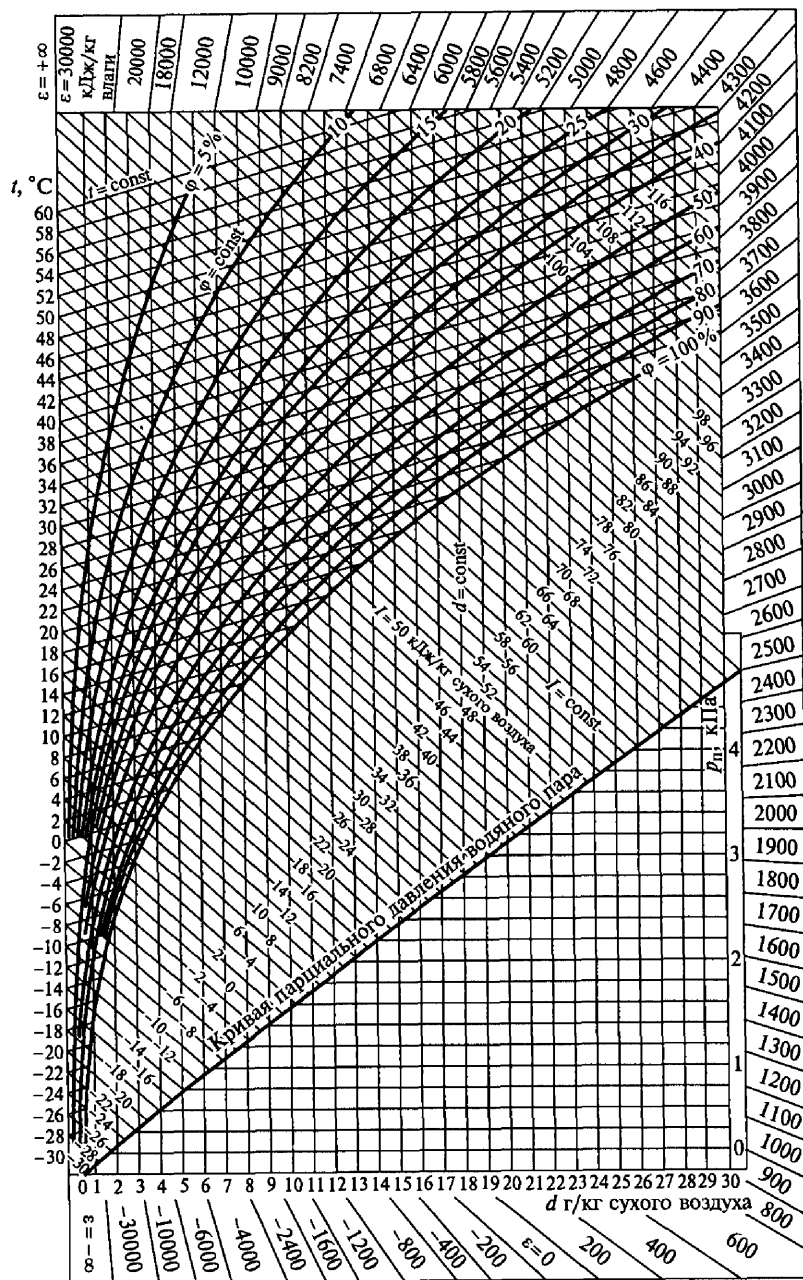
Рис. 6.1. I — d -диаграмма влажного воздуха
