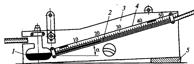
Рис. 10.2. Наклонный напорометр:
