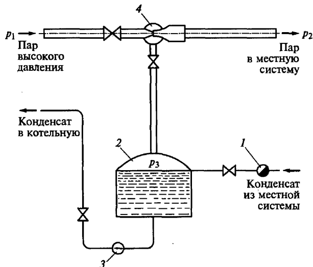
Рис. 11.5. Схема установки инжектора:
