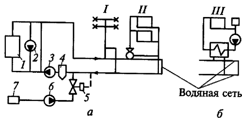
Рис. 1.11. Структурная схема районного теплоснабжения от водогрейной котельной:
