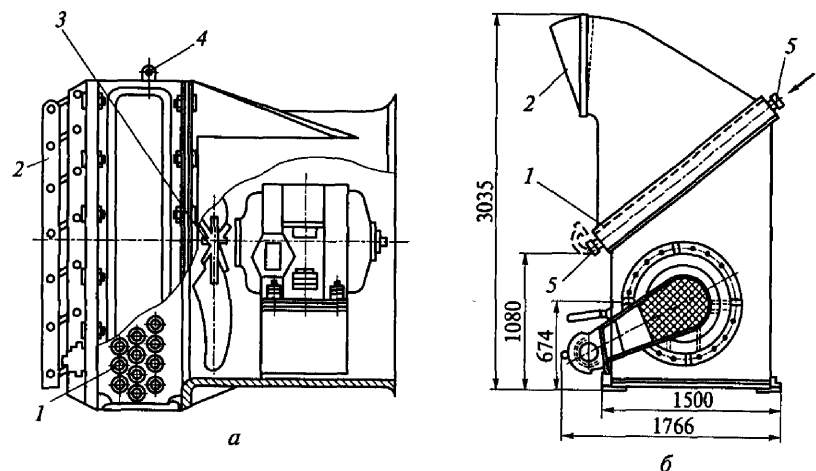
Рис. 3.22. Подвесные и напольные воздушные отопительные агрегаты:
