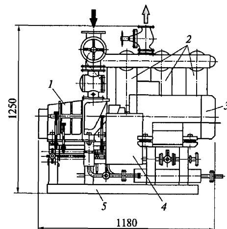
Рис. 9.16. Общий вид аммиачного компрессорного агрегата 2А50Б-7:
