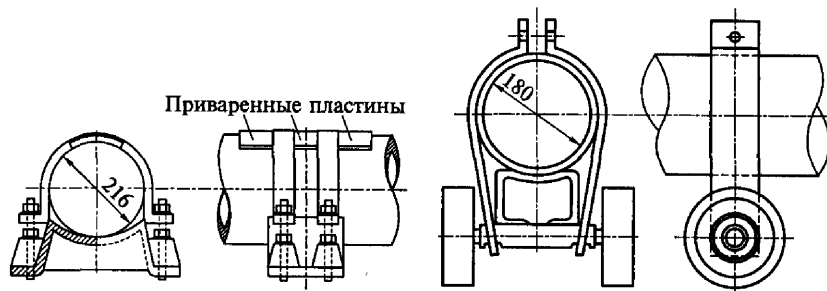
Рис. 1.18. Неподвижная опора
