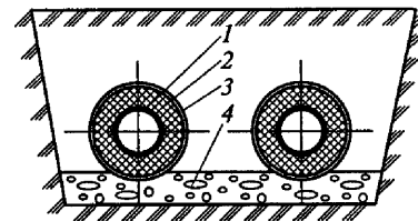
Рис. 1.15. Бесканальная прокладка теплопровода в битумоперлитной изоляции:
