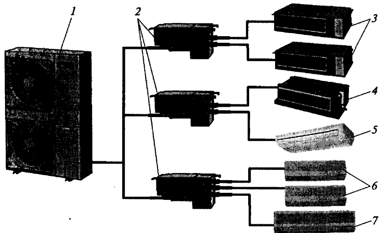
Рис. 9.15. Система кондиционирования Super Multi Plus:
