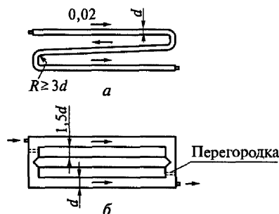
Рис. 4.1. Регистры из стальных труб: а — диаметром 32...40 мм; б — диаметром 76...109 мм
