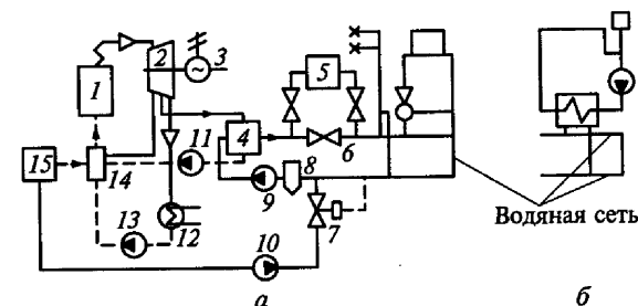
Рис. 1.13. Структурная схема теплофикации:
