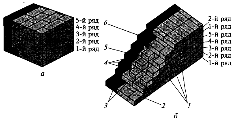
Рис. 2.1. Конструкция кладки из утолщенного кирпича «Термолюкс®»: а — фрагмент кладки; б — вертикальный разрез; 1 — поперечные вертикальные швы; 2 — внутренняя верста; 3 — продольные вертикальные швы; 4 — ложковые кирпичи; 5 — наружная верста; 6 — лицевой кирпич
