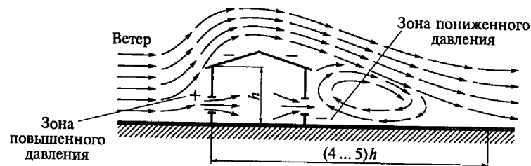
Рис. 7.4. Движение воздушных потоков при обтекании здания в ветреную погоду
