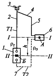
Рис. 3.7. Схема, поясняющая естественную циркуляцию теплоносителя в системе водяного отопления: 1 — котел; 2 — главный стояк; 3 — расширительный бак; 4 — магистраль горячей воды; 5 — отопительный стояк; 6 — отопительный прибор; 7 — магистраль охлажденной воды; \rho_r , \rho_0 — плотности соответственно горячей и охлажденной воды; A — центр охлаждения; B — центр нагревания
