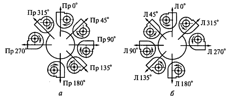
Рис. 8.1. Положения корпусов вентиляторов правого (а) и левого (б) вращений
