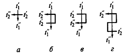
Рис. 1.8. Варианты перекрестных токов в теплообменниках: а — одноходовый; б, в — двухходовых; г — трехходовый
