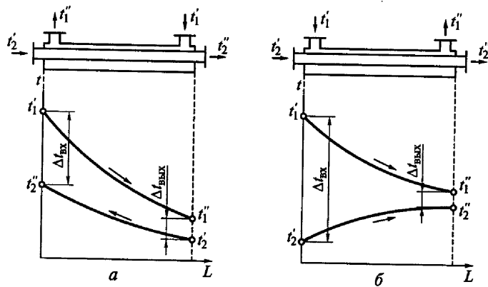
Рис. 1.7. Схема движения и график изменения температур теплоносителей: а — противоток; б — прямоток
