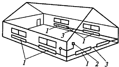
Рис. 3.31. Эскиз размещения электроконвекторов в жилом помещении: 1 — электроконвекторы; 2 — термостат; 3 — электрические провода
