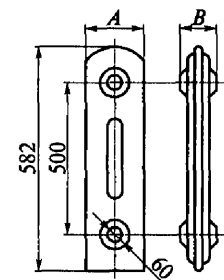
Рис. 4.2. Секция чугунных радиаторов
