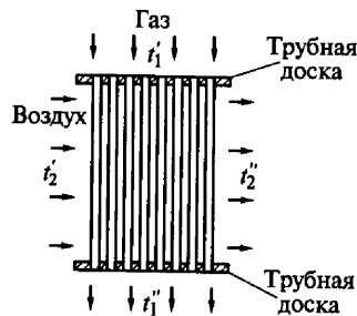
Рис. 1.10. Схема одноходового воздухоподогревателя
