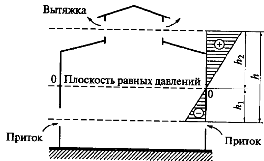
Рис. 7.3. Схема распределения давления воздуха при естественной вентиляции в здании
