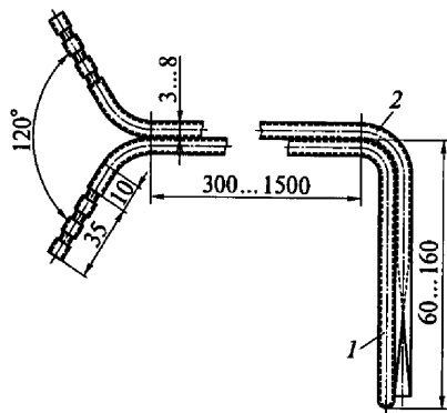
Рис. 10.3. Пневмометрическая трубка
