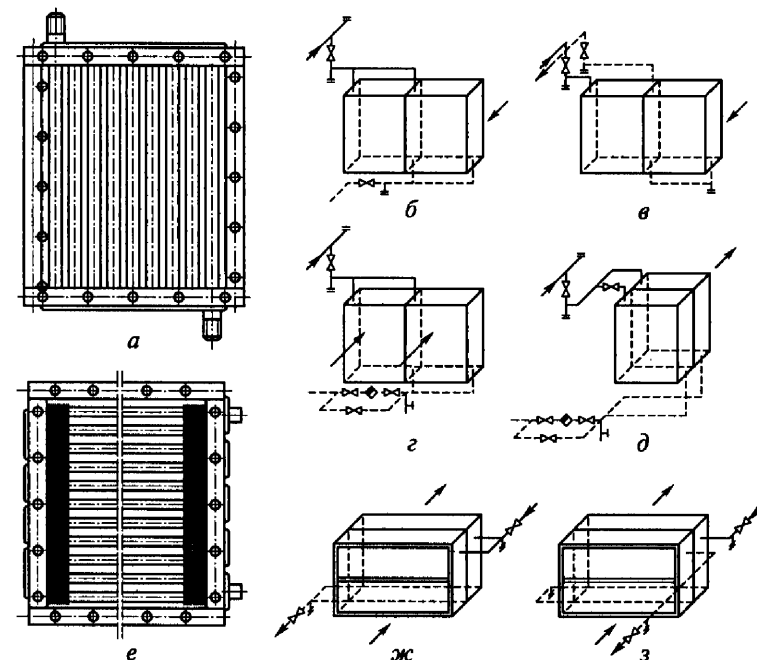
Рис. 8.4. Калориферы и схемы их обвязок:
