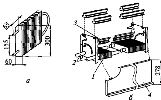
Рис. 4.5. Конвекторы:
