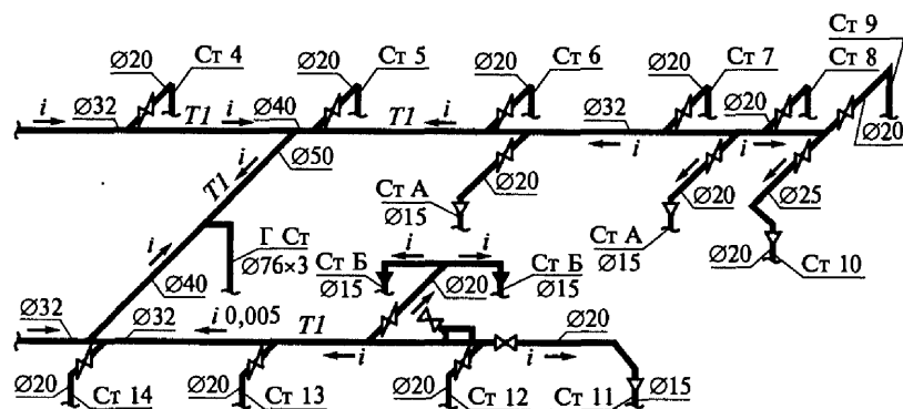
Рис. 3.5. План чердака жилого здания с верхней разводящей сетью трубопроводов отопления (a) и аксонометрическая схема верхней разводки (б)
