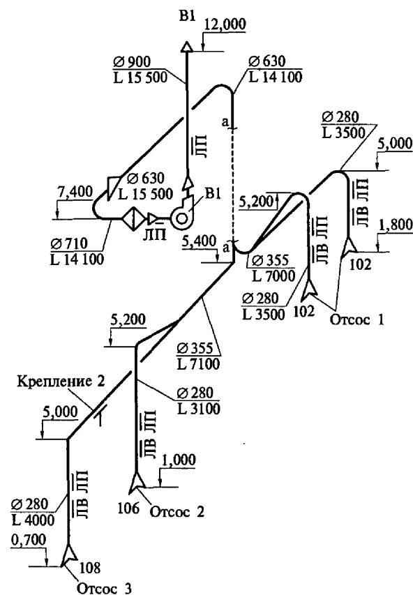
Рис. 12.2. Аксонометрическая схема вытяжной вентиляции производственного здания
