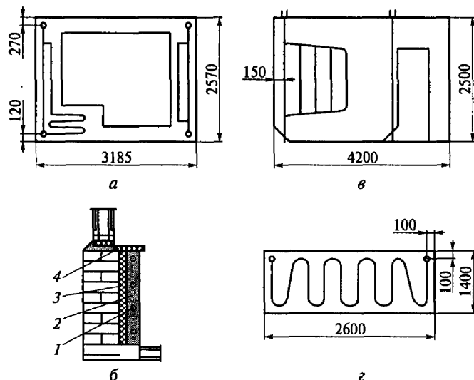
Рис. 4.6. Бетонные отопительные панели:
