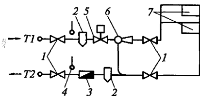
Рис. 1.1. Схема индивидуального теплового пункта:
