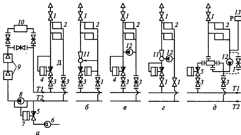
Рис. 1.14. Варианты схем присоединения местных систем отопления и горячего водоснабжения в двухтрубных водяных системах:
