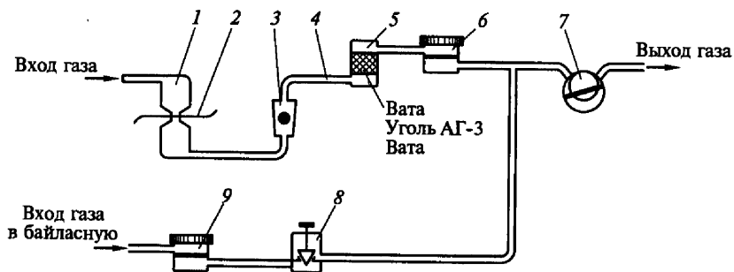
Рис. 10.8. Газовая схема универсального ленточного фотометра ФЛ 5501М:
