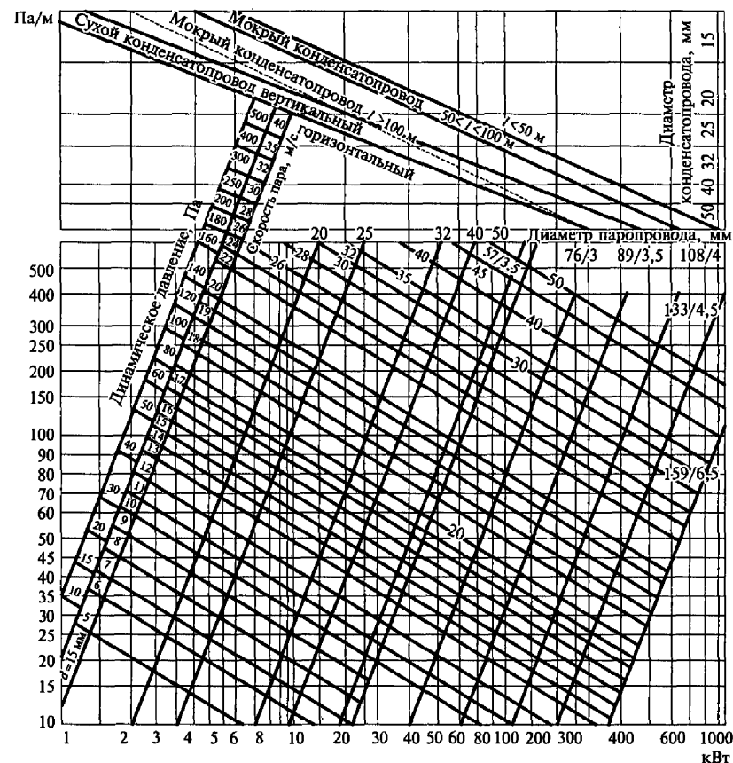
Рис. 3.20. Номограмма для расчета диаметров паропроводов и самотечных конденсатопроводов
