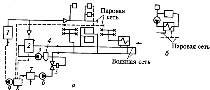
Рис. 1.12. Структурная схема районного теплоснабжения от паровой котельной:
