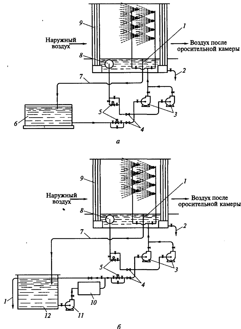
Рис. 9.8. Схемы устройства водяной сети кондиционера:
