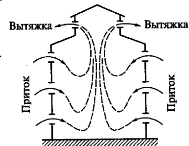
Рис. 7.1. Движение воздушных потоков при естественной вентиляции здания
