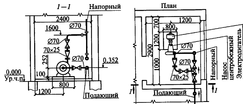
Рис. 3.12. Разрез и план помещения насосной установки для повышения напора в системе отопления многоэтажного здания
