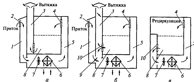
Рис. 3.21. Схемы систем воздушного отопления:
