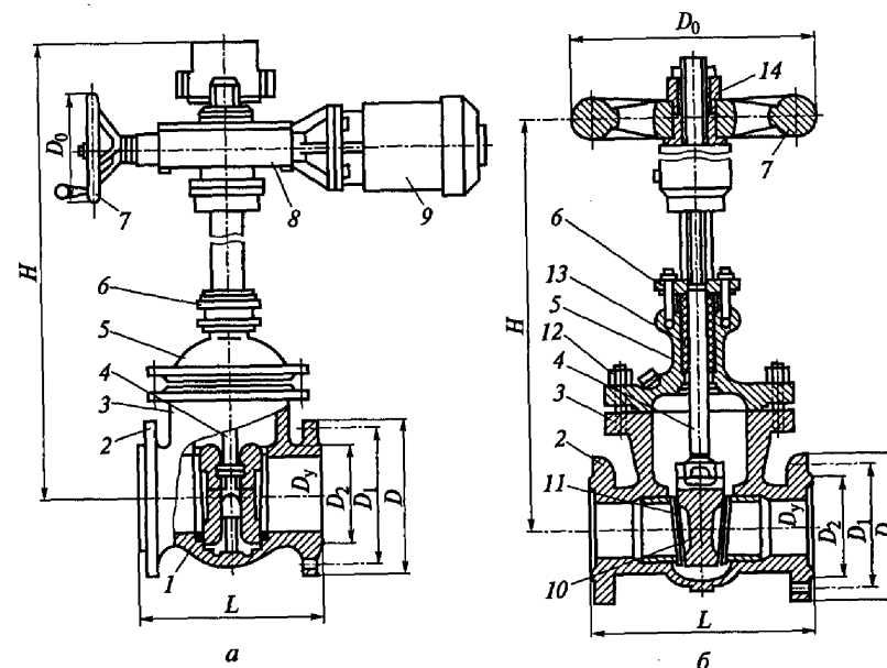
Рис. 5.1. Задвижки:
