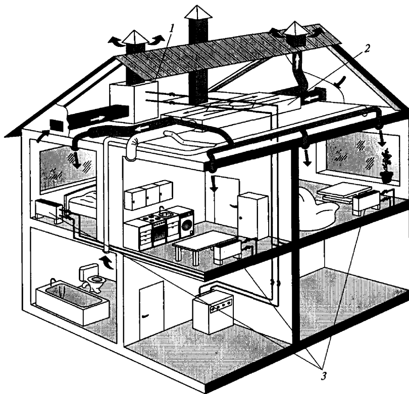
Рис. 9.20. Система кондиционирования воздуха на базе чиллера и фанкойлов:
