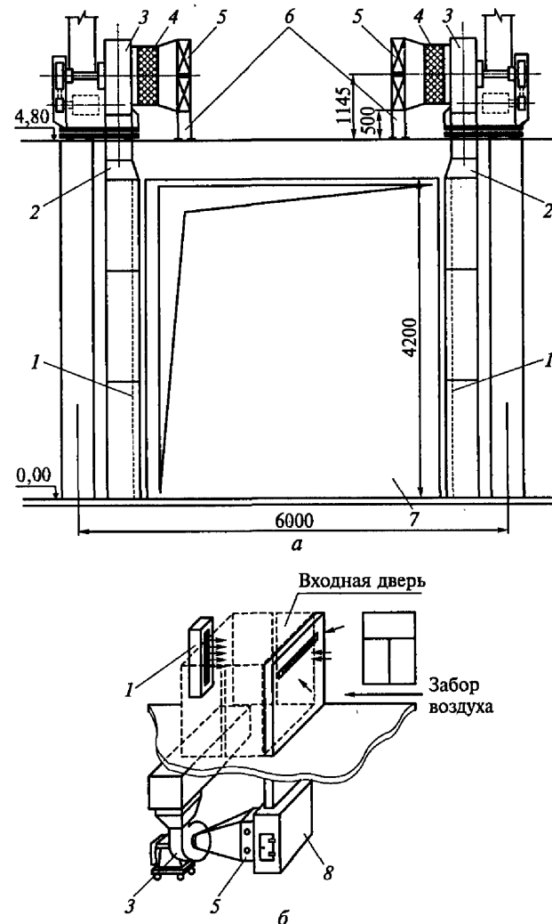
Рис. 3.23. Способы размещения оборудования тепловых воздушных завес: а — в промышленных зданиях; б — в общественных зданиях; 1 — воздухоподразделительная щель; 2 — конфузор; 3 — вентилятор; 4 — мягкая вставка; 5 — калорифер; 6 — подставка; 7 — ворота; 8 — секция обслуживания
