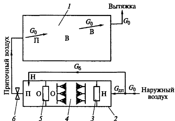
Рис. 9.4. Схема системы кондиционирования воздуха в летнее время с использованием адиабатического процесса обработки и подмешивания части наружного воздуха в зоне за оросительной камерой (номера позиций соответствуют рис. 9.2)
