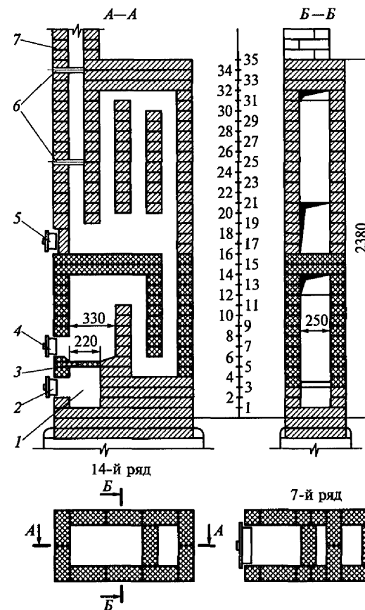
Рис. 3.26. Конструкция толстостенной печи ОПЗ-3:
