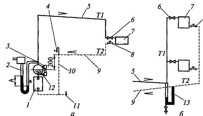
Рис. 3.16. Система парового отопления низкого давления:
