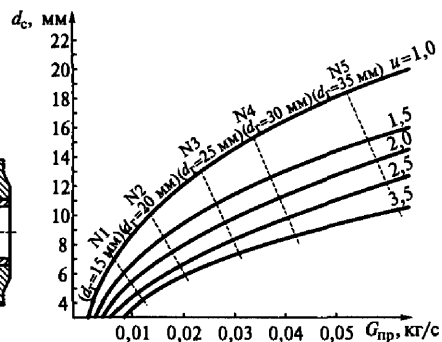
Рис. 3.14. Номограмма для выбора элеватора
