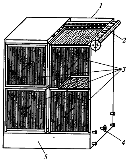
Рис. 11.1. Камера с волнисто-параллельной орошаемой насадкой: 1 — корпус; 2 — коллектор для раздачи воды; 3 — кассеты; 4 — выходной патрубок; 5 — поддон
