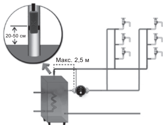
Рис. 43 Насос COMFORT BA(X), BT(X) со встроенный датчиком температуры
