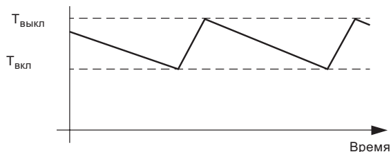
Рис. 41 Режим контроля температуры
