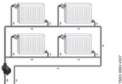
Рис. 4 Однотрубная система отопления
