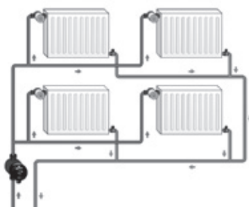
Рис. 5 Двухтрубная система отопления
