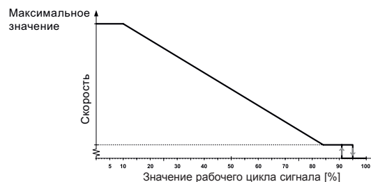
Рис. 15 Профиль управляющего ШИМ-сигнала в ALPHA1 L
