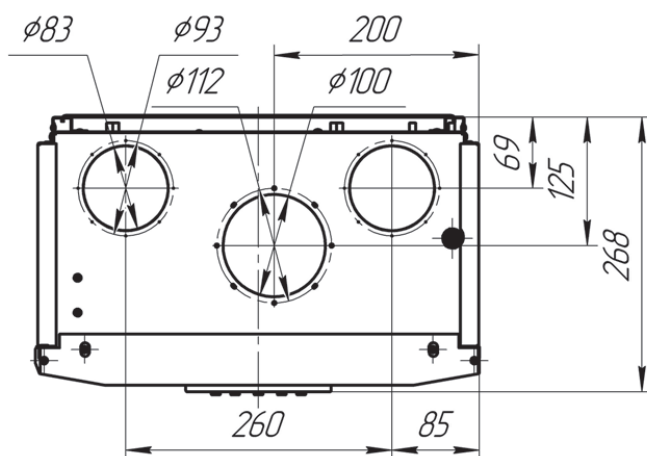
Вид сверху
