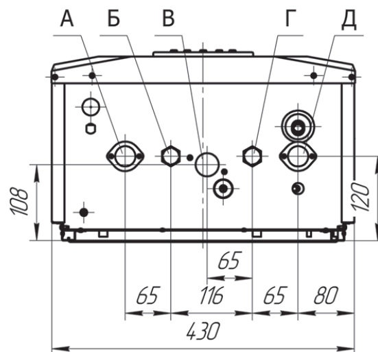
Вид снизу
