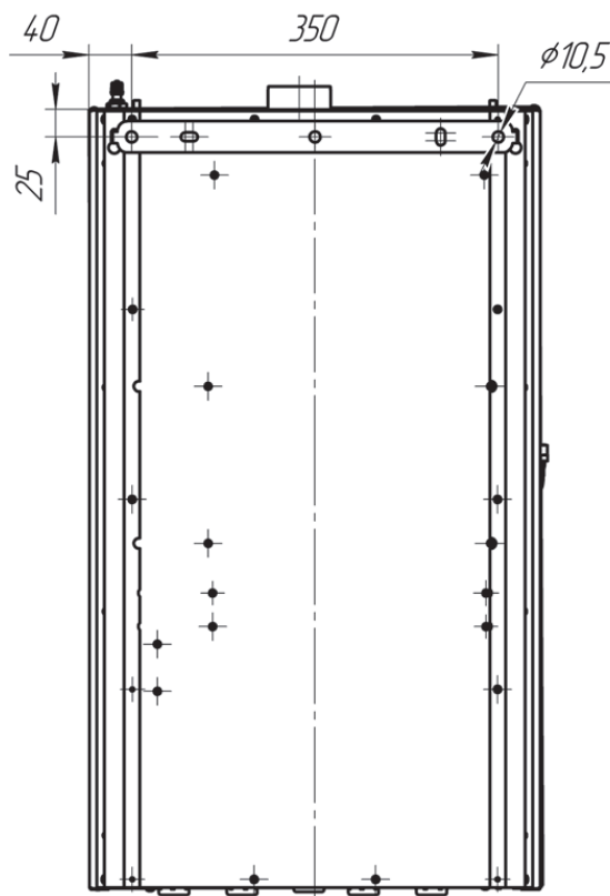
Вид снизу
