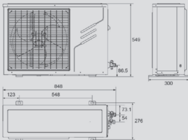
Габаритные размеры для моделей MCL-03
