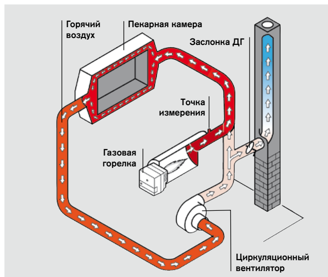
Печь с прямым горением
