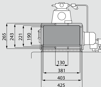
Система забора воздуха, вид снизу
