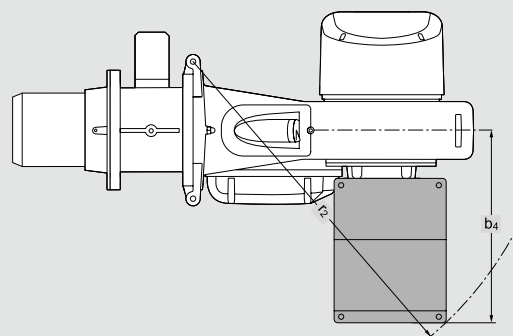
Частотный преобразователь (Серия WM 30/3)
