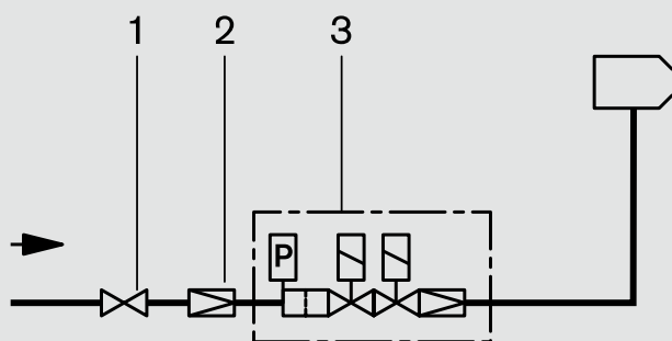
Расположение газовой арматуры при давлении подключения до 300 мбар
