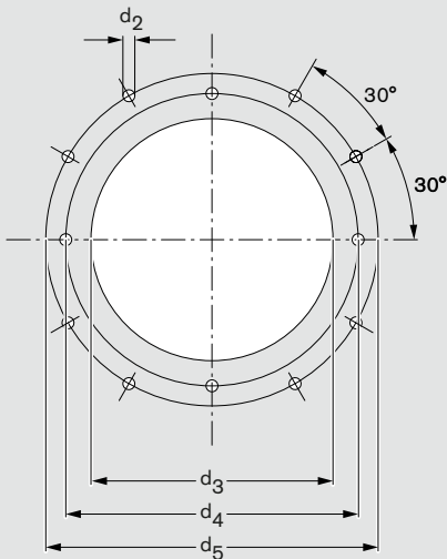
Отверстия в плите котла
