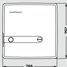
Габаритные размеры горелки типа WL5-B, WL 5-B-H и WL5/2-B, исполнение стандартное (размеры в мм)
