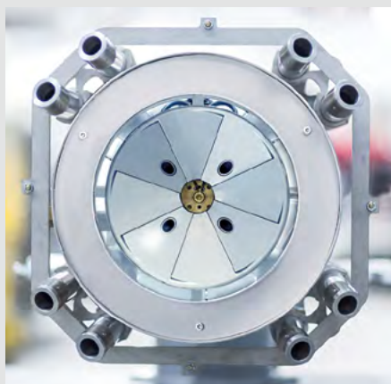
Газовое смесительное устройство исп. multiflam®
