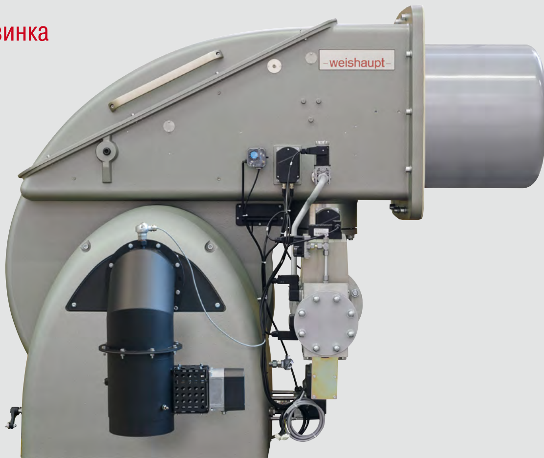
Принципиальная конструкция системы рециркуляции дымовых газов с WKmono 80
