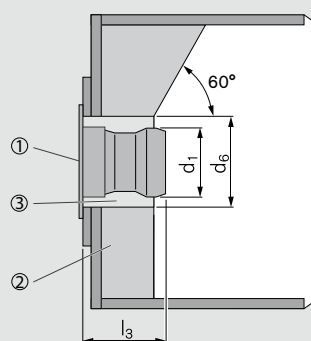
Подготовка теплогенератора
