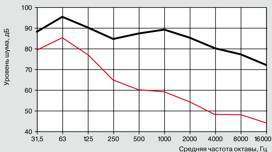
Измерение уровня шума – пример 2
