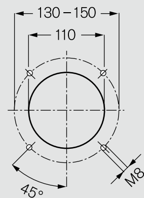
Размеры отверстий монтажной плиты
