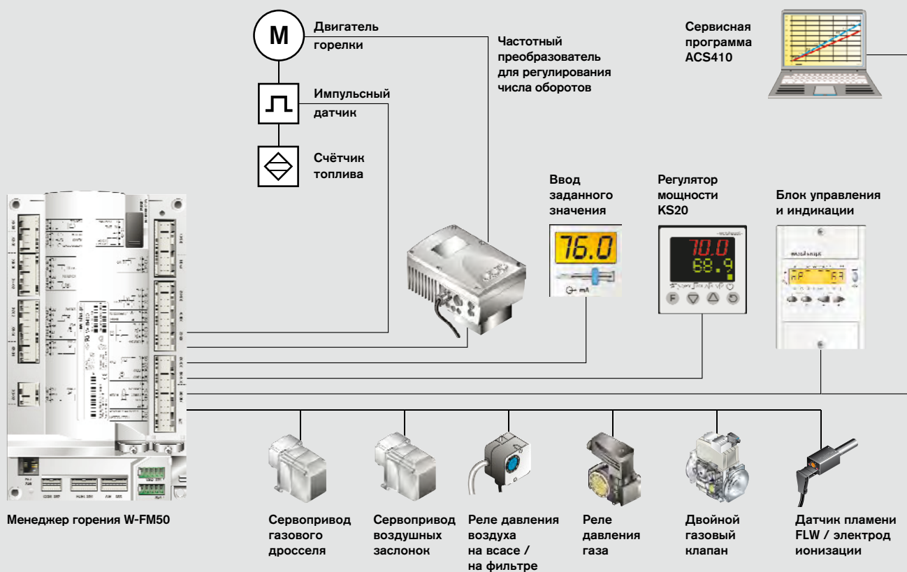
Горелка со встроенным цифровым менеджером горения
