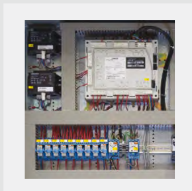
Менеджер горения W-FM100 или W-FM200 в шкафу управления
