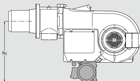
Встроенный топливный насос (Серия WM 30/3)
