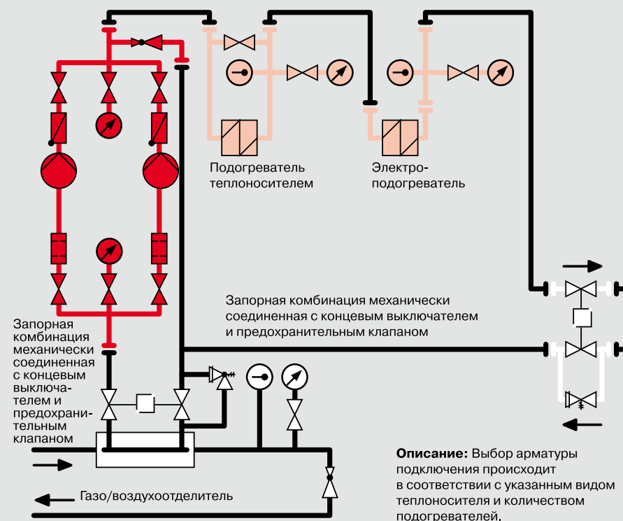
Станция подогрева (теплоносителем)
