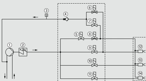
Исполнение (ZM)-T. Топливо S
