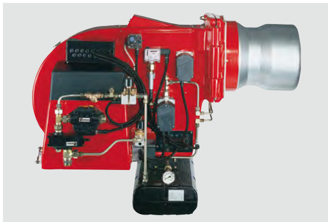
Мазутная горелка RMS 60/2-A с цифровым менеджером горения
