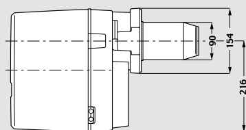
Габаритные размеры горелки типа WL5-B, WL 5-B-H и WL5/2-B, исполнение стандартное (размеры в мм)
