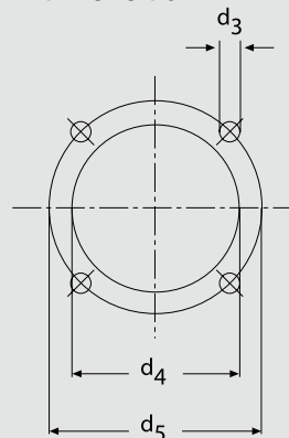
Отверстия в плите котла
