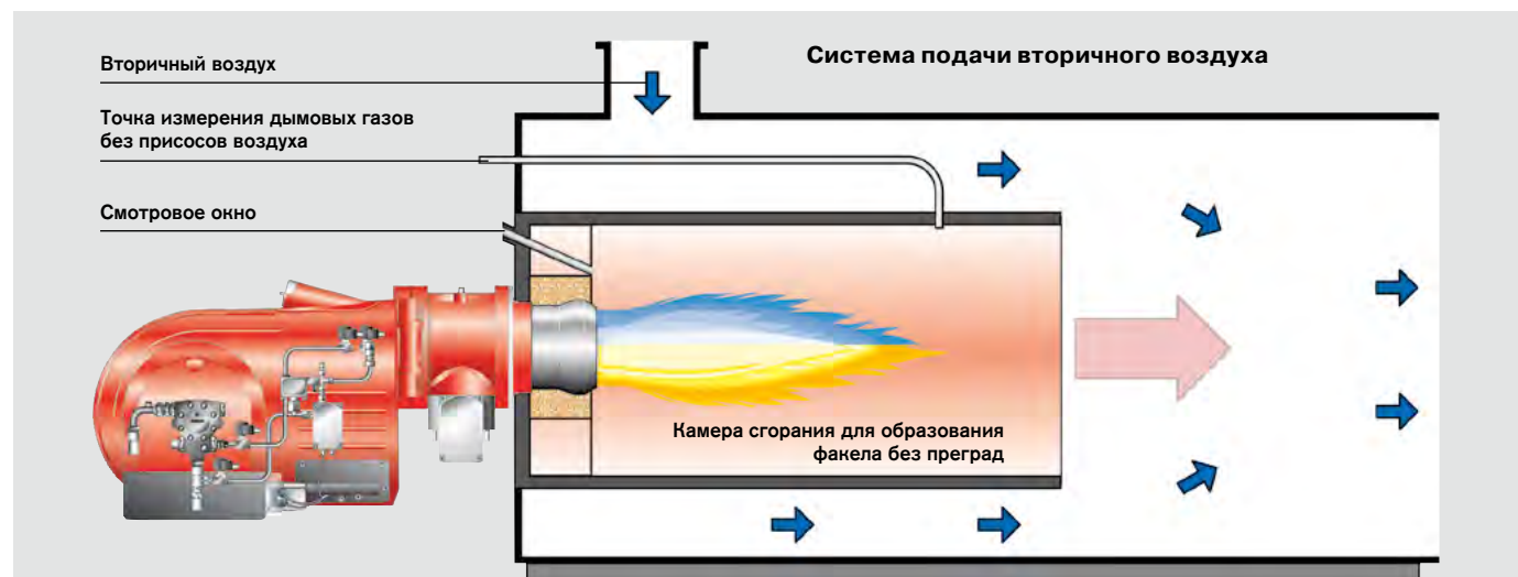
Печь с непрямым горением (теплообменники)
