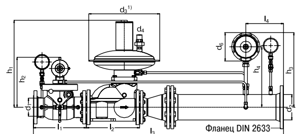
Рис. 4 – тип 9
