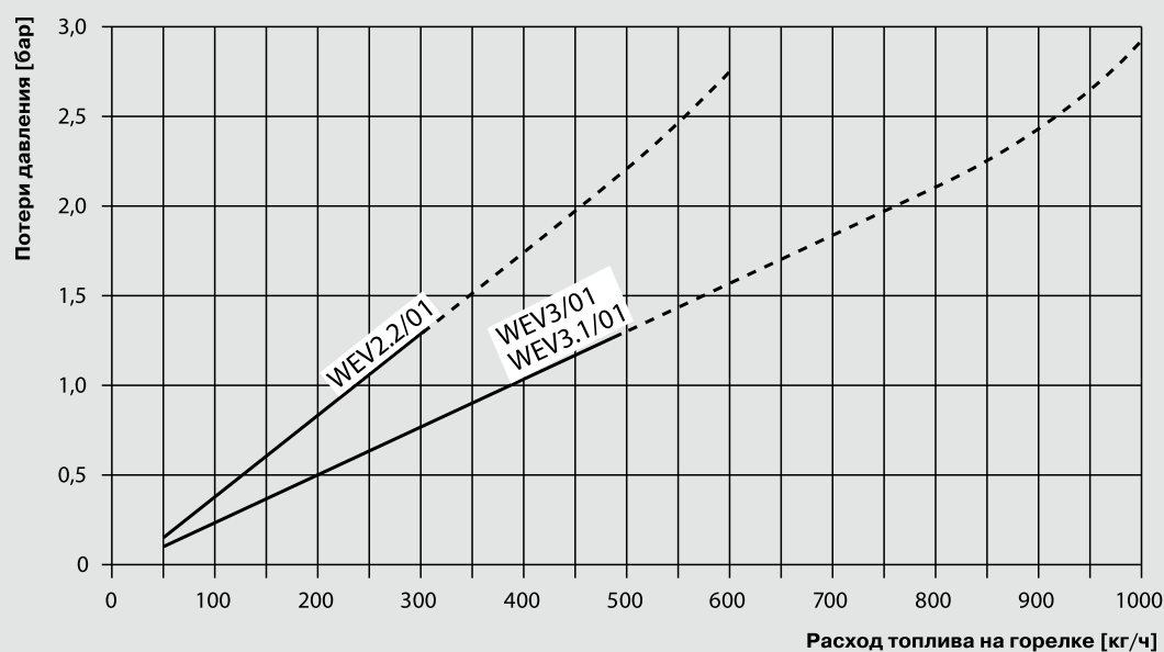
Потери давления WEV...
