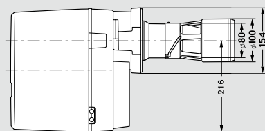
Габаритные размеры горелок типа WL5-B-H, исполнение 2LN, (размеры в мм)
