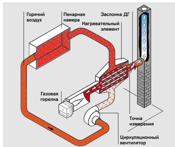
Печь с непрямым горением (теплообменники)
