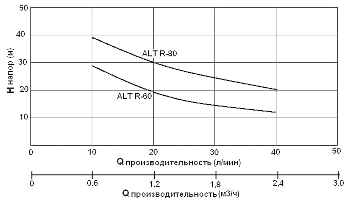
ДИАГРАММА НАПОРНО-РАСХОДНЫХ ХАРАКТЕРИСТИК
