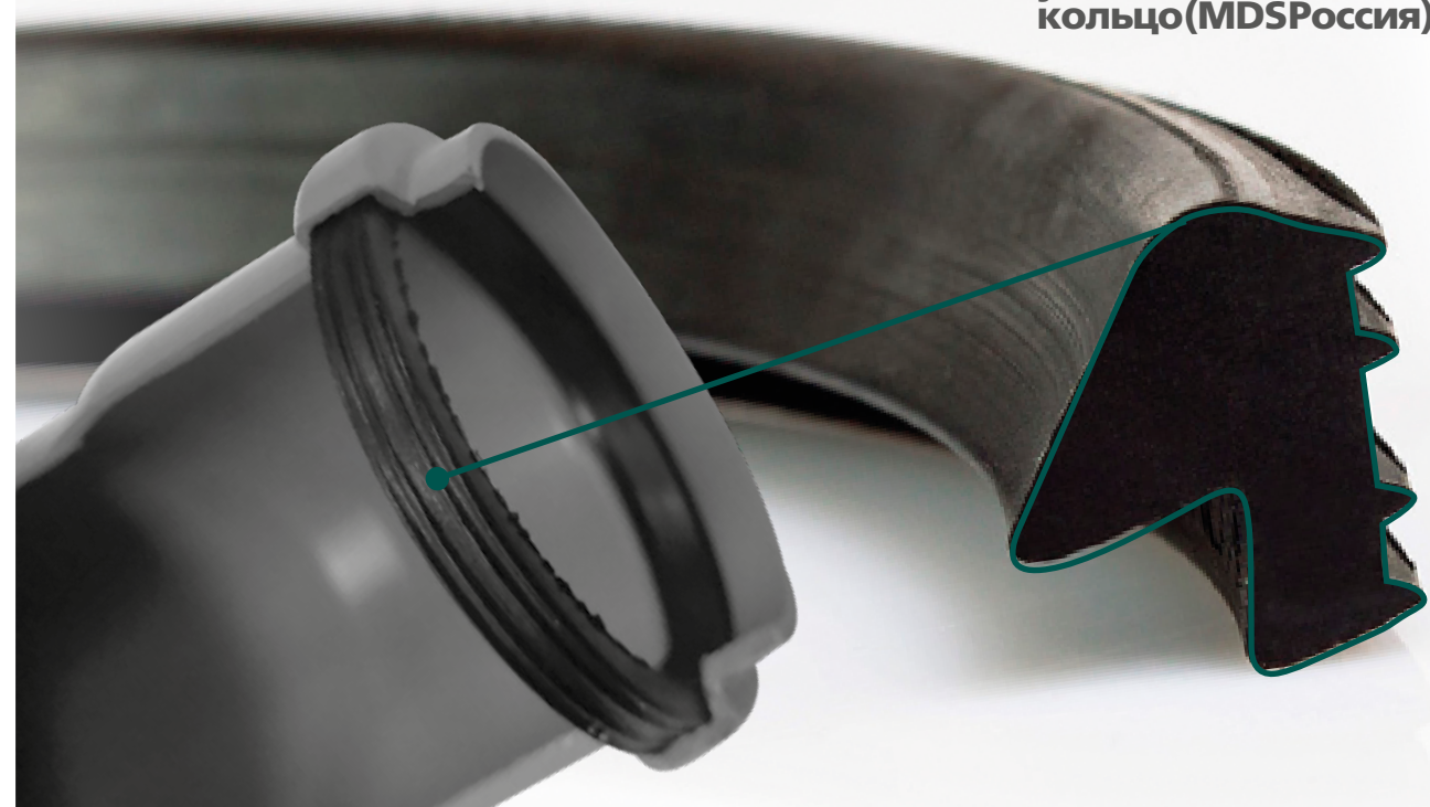
Однолепестковое уплотнительное кольцо (MDSРоссия)
