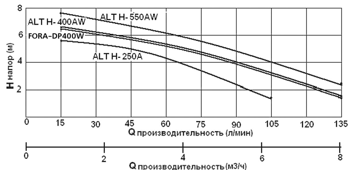
ДИАГРАММА НАПОРНО-РАСХОДНЫХ ХАРАКТЕРИСТИК
