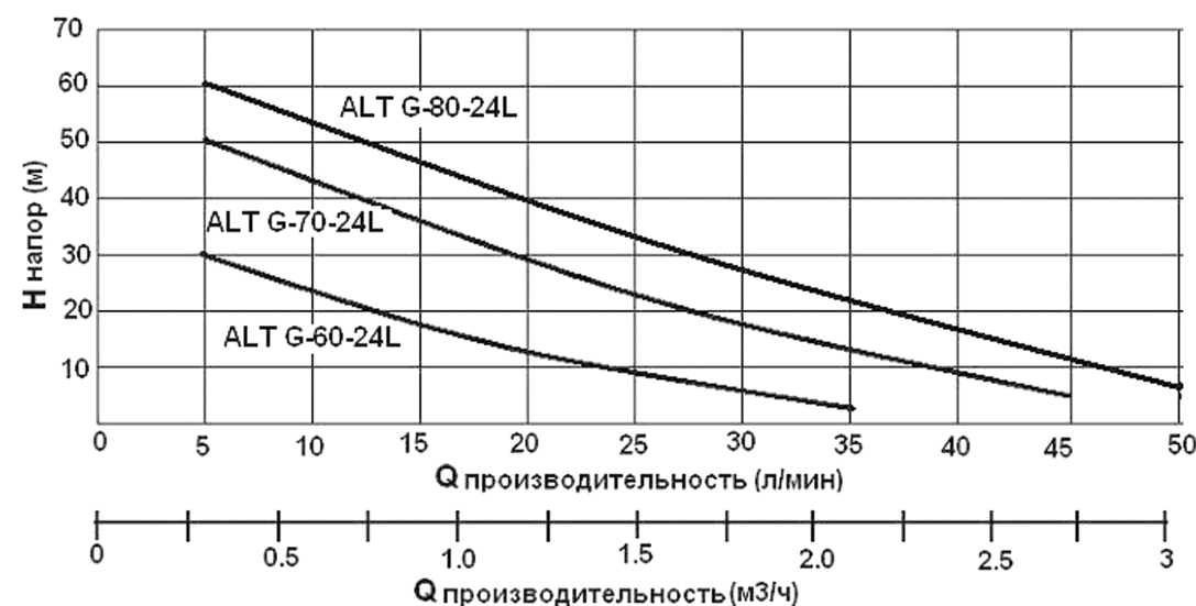
ДИАГРАММА НАПОРНО-РАСХОДНЫХ ХАРАКТЕРИСТИК
