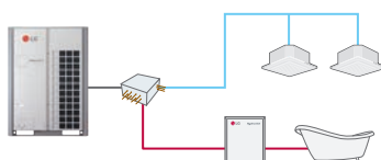
Блок рекуперации теплоты (энергоэффективность)
