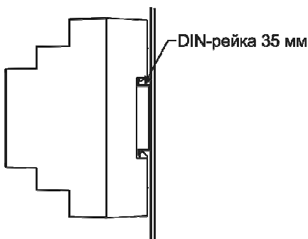
Рисунок 2 – Установка изделия
