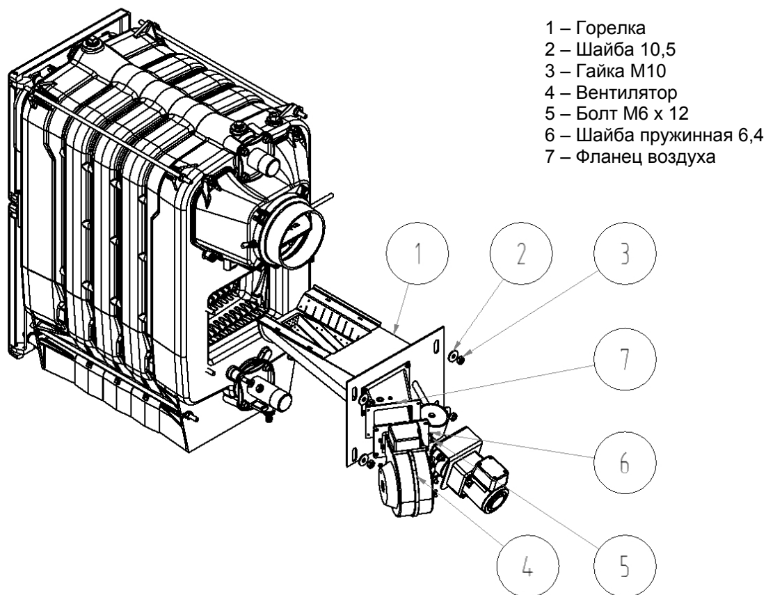
Рис. № 10 Монтаж горелки
