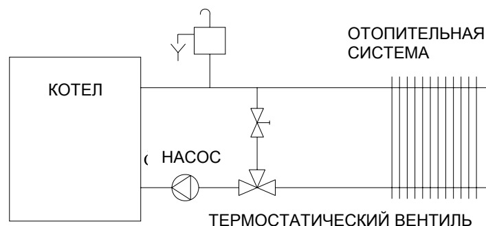
Рис. no. 8 Рекомендуемая схема подключения котла к отопительной системе
