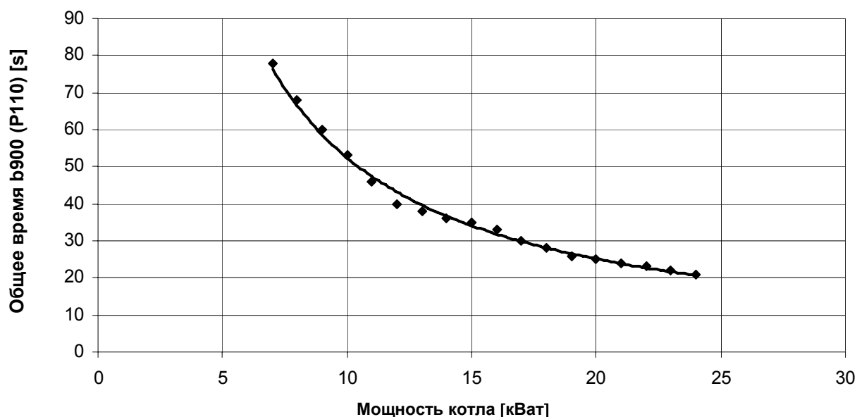
Рис. no. 22 Граф зависимости мощности котла на времени для прогорания топлива при одинаковом времени для подачи топлива (5 s) для котла VIADRUS HERCULES ECO - 5 секций
