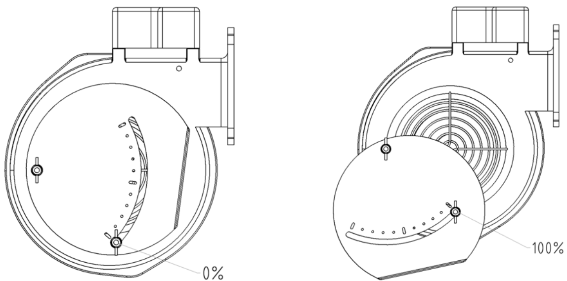
Рис. no. 21 Клапан дроссельный вентилятора
