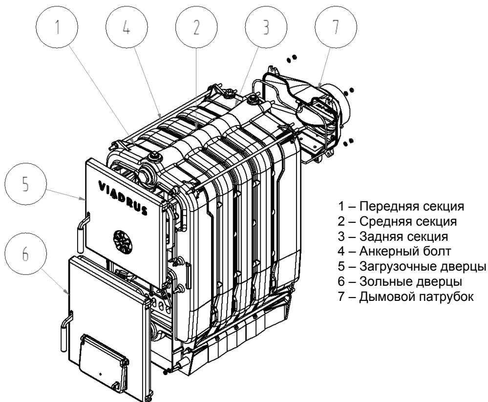
Рис. no. 3 Чугунный корпус котла VIADRUS HERCULES ECO
