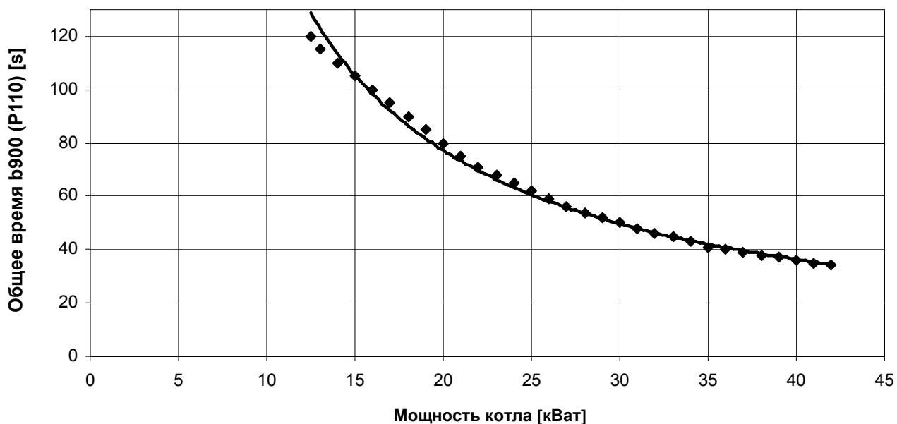
Рис. но. 23 Граф зависимости мощности котла на времени для прогорания топлива при одинаковом времени для подачи топлива (10 s) для котла VIADRUS HERCULES ECO - 10 секций
