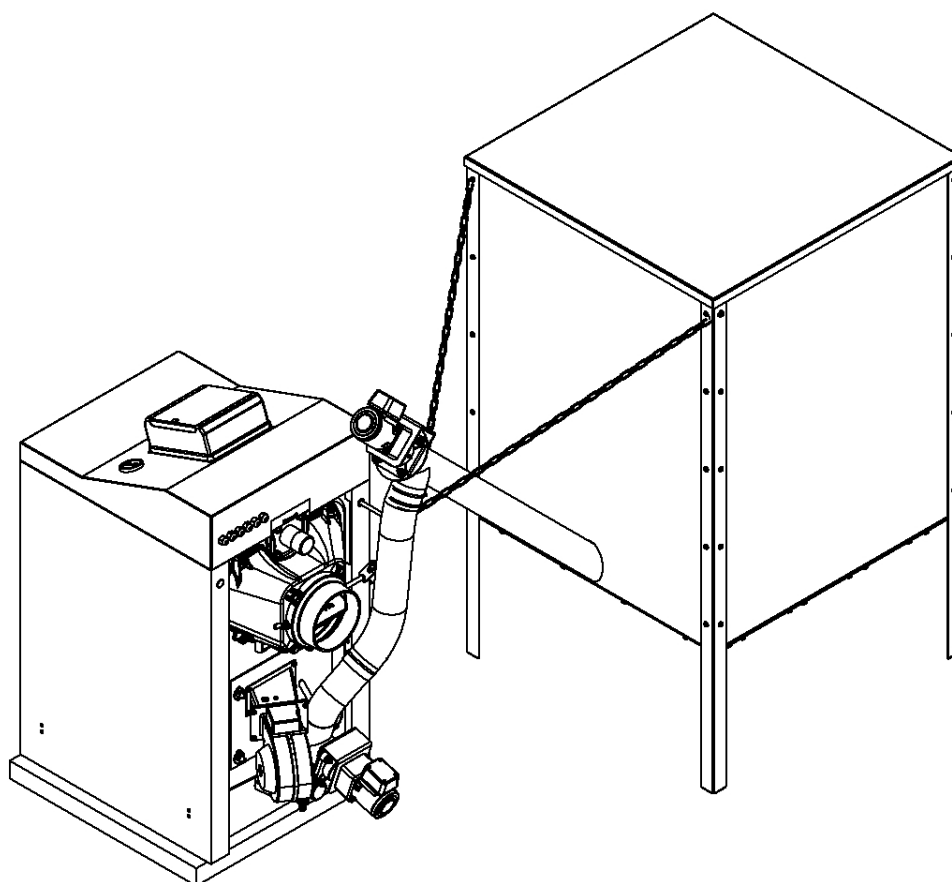
Рис. но. 2 Вид котла сзади VIADRUS HERCULES ECO с бункером топлива – левая версия
