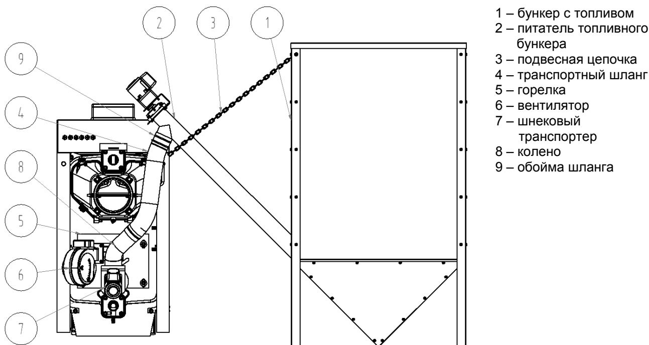
Рис. no. 15 Монтаж топки котла VIADRUS HERCULES ECO
