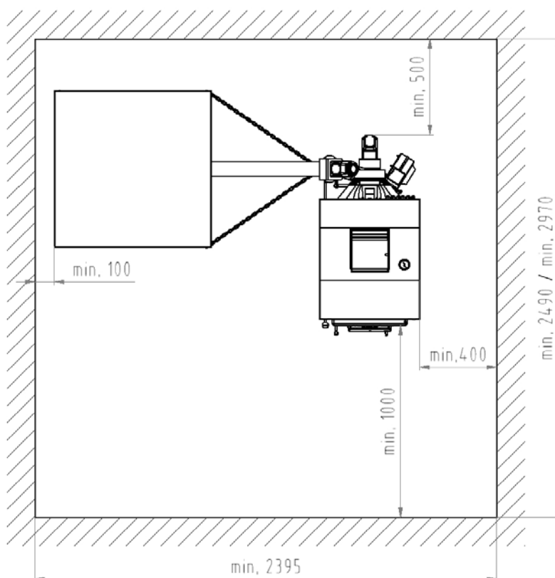
Рис. no. 7 Расположение котла VIADRUS HERCULES ECO в котельной (цифра за знаком деления относится к версии с 10 секциями)
