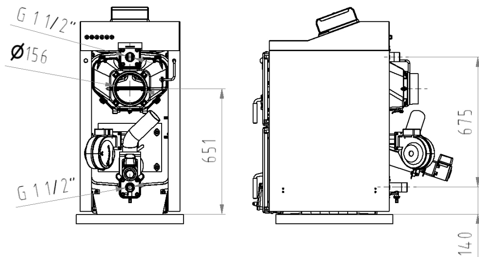
Рис. no. 9 Присоединительные размеры котла VIADRUS HERCULES ECO
