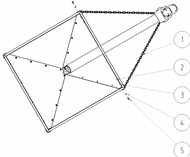
Рис.№ 18 Монтаж подвесных цепочек к топливному бункеру
