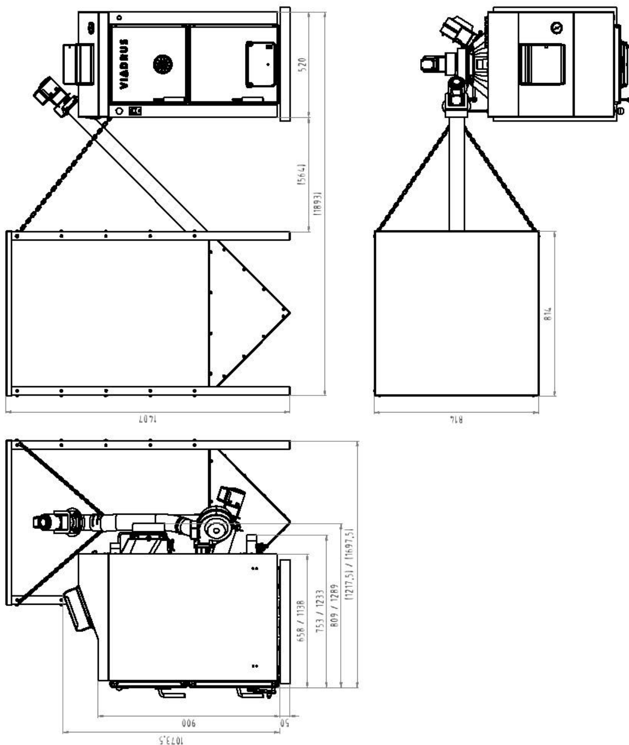
Рис. no. 4 Размеры котла VIADRUS HERCULES ECO (значения за знаком деления относятся к версии с 10 сек)
