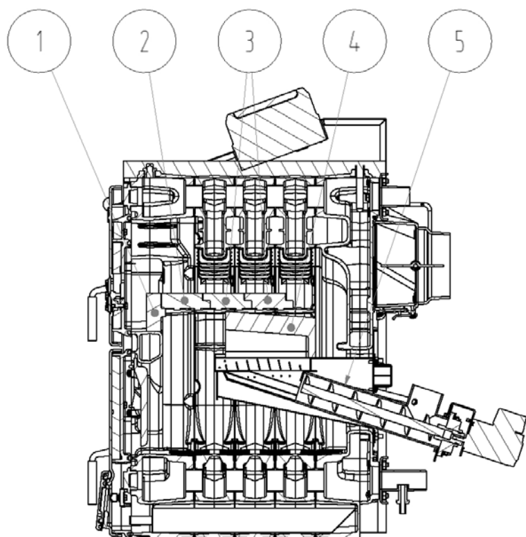
Рис. no. 13 Укладка керамических досок в корпус котла с 5 секциями
