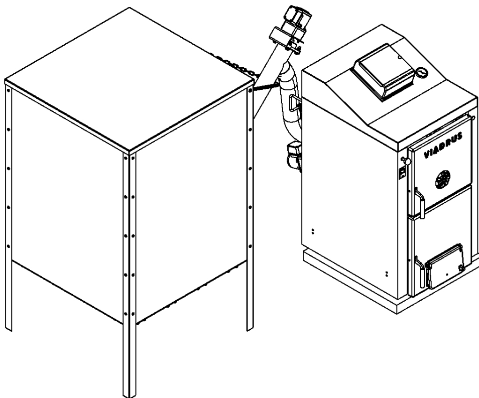
Рис. но. 1 Вид котла спереди VIADRUS HERCULES ECO с бункером топлива – левая версия
