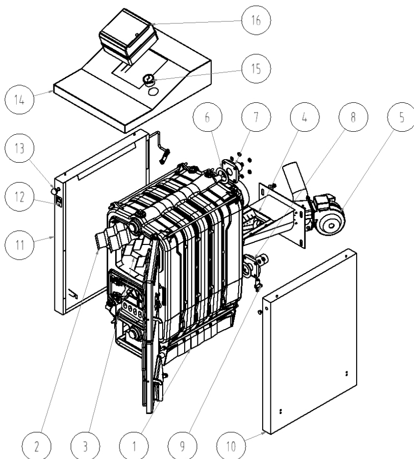
Рис. no. 5 Котел VIADRUS HERCULES ECO
