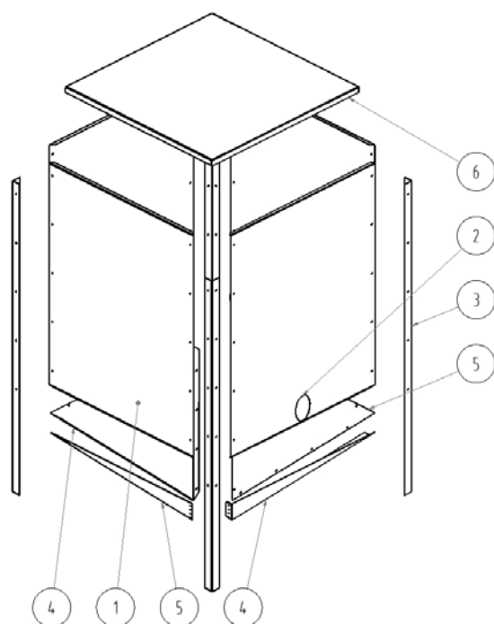
Рис. no. 17 Монтаж топливного бункера
