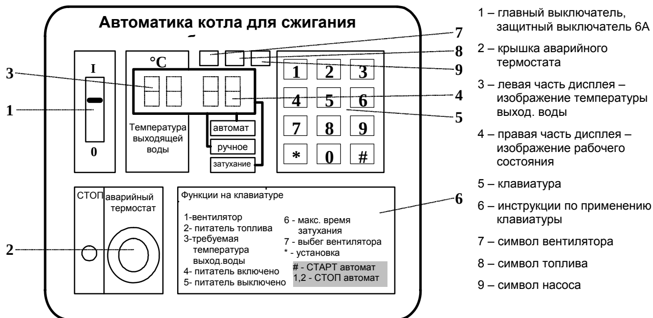
Рис. no. 19 Панель управления регулятора MONEX
