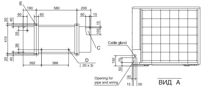
ВИД А
