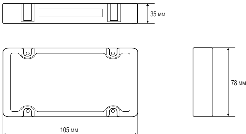
PQDSB (модуль внешнего сигнала)
