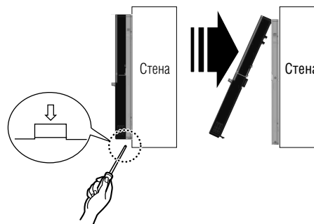
<Последовательность демонтажа>
