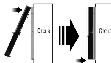
<Последовательность демонтажа>
